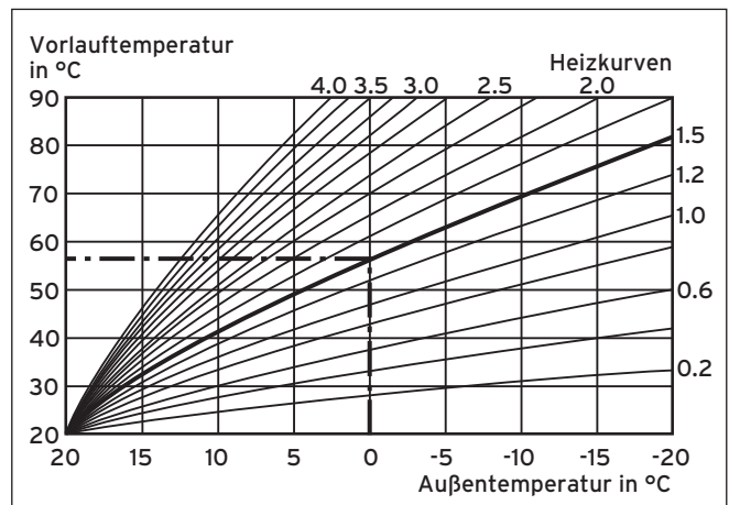
Abb. 13.1 Diagramm mit Heizkurven
