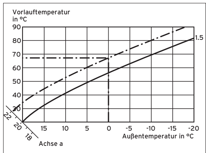
Abb. 13.2 Parallelverschiebung der Heizkurve
