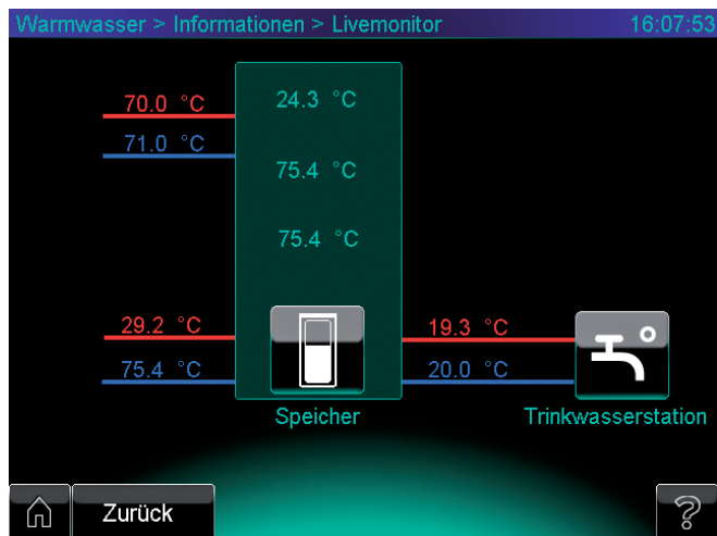
Abb. 7.2 Anlagenübersicht Warmwasserkreis/Pufferspeicher
