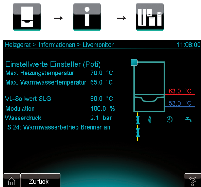
Abb. 7.5 Anlagenübersicht Spitzenlastgerät
