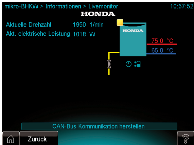
Abb. 7.6 Anlagenübersicht KWK-Modul
