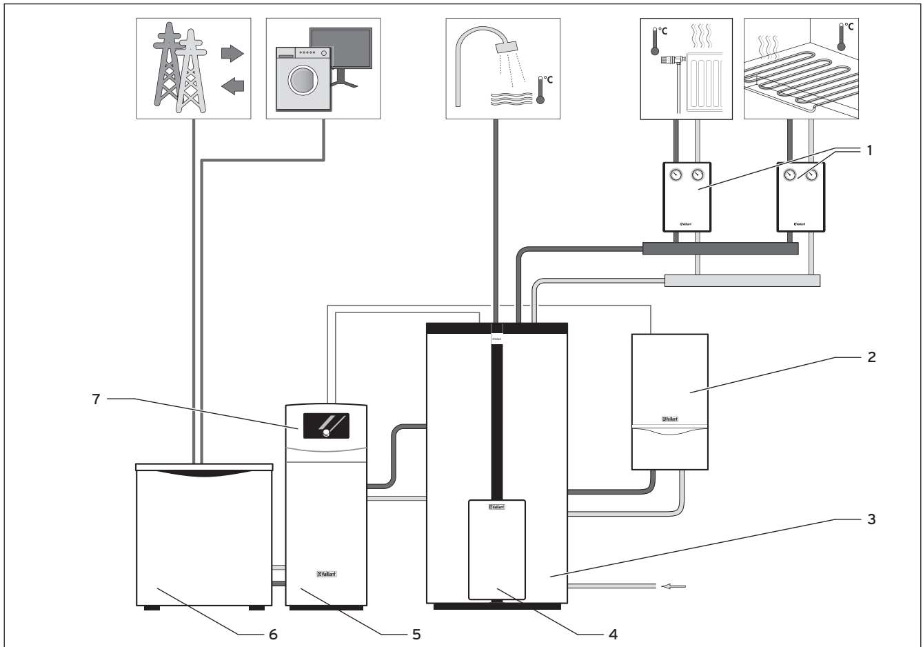
Abb. 4.1 Prinzipdarstellung System ecoPOWER 1.0
