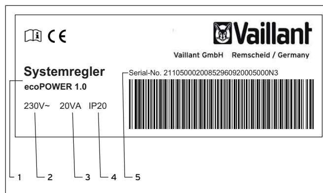
Abb. 1.2 Typenschild Systemregler
