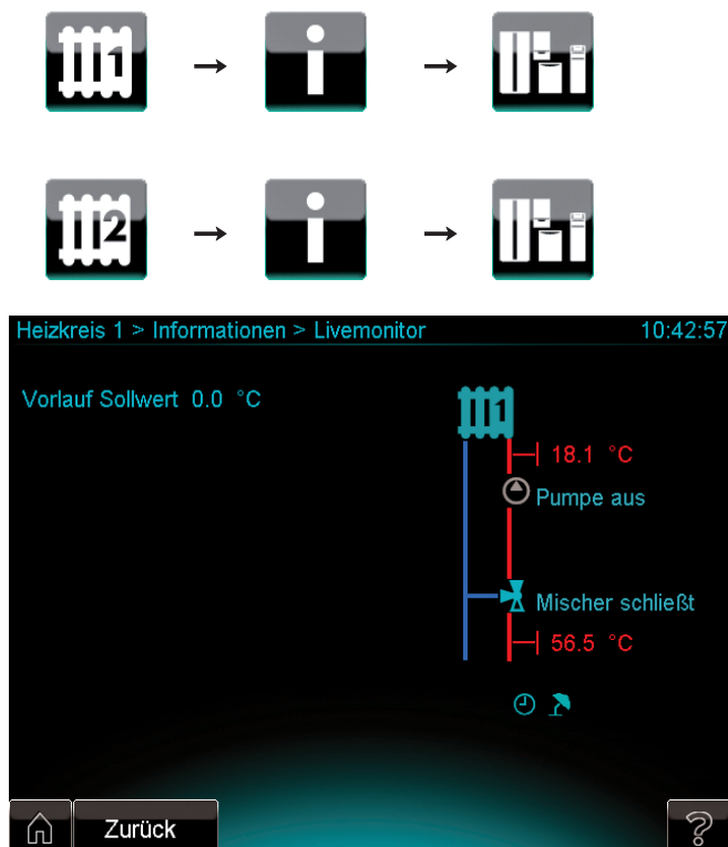
Abb. 7.4 Anlagenübersicht Heizkreis 1
