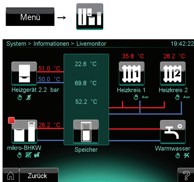
Abb. 7.1 Anzeige Anlagenübersicht/Livemonitor
