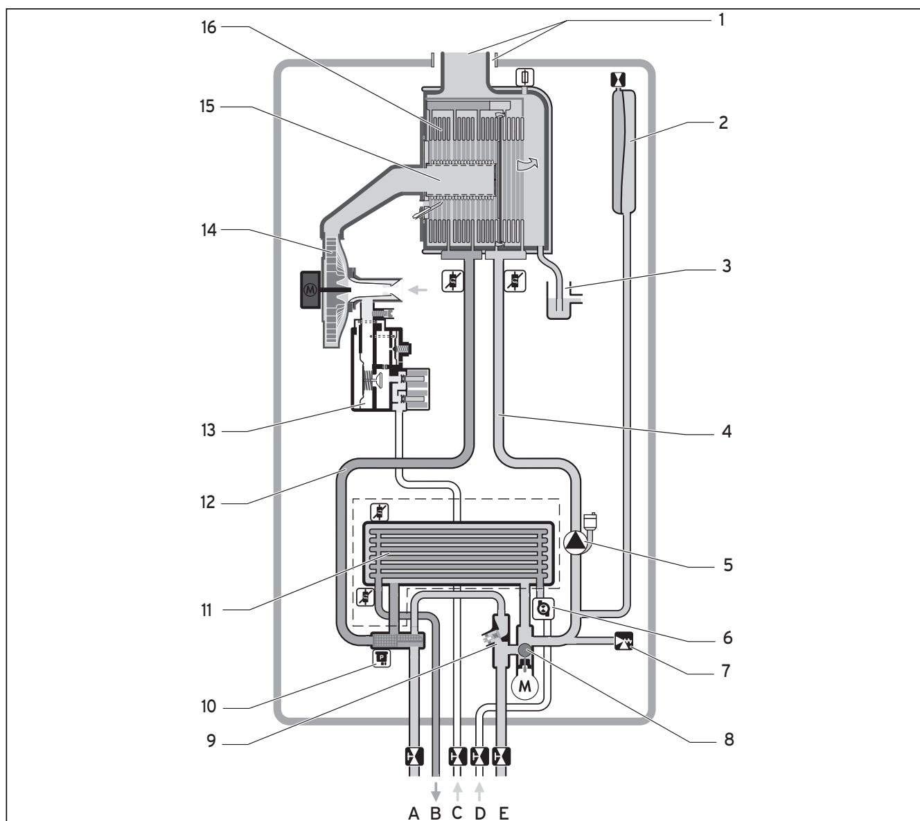
Abb. 4.1 Funktionsschema ecoTEC VCW plus
