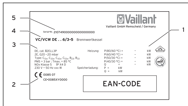
Abb. 1.1 Typenschild
