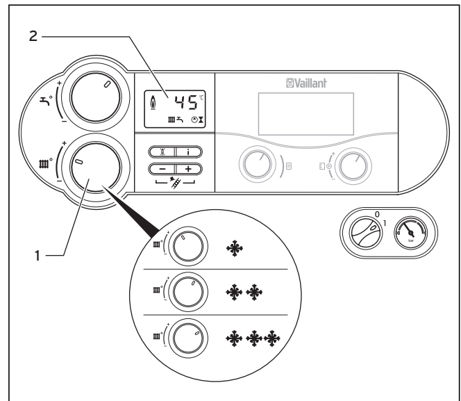
Abb. 5.11 Vorlauftemperatur einstellen ohne Regelgerät
