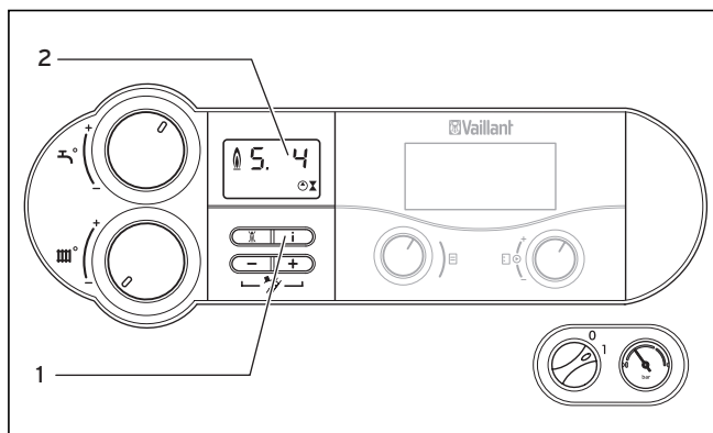
Abb. 5.17 Statusanzeigen
