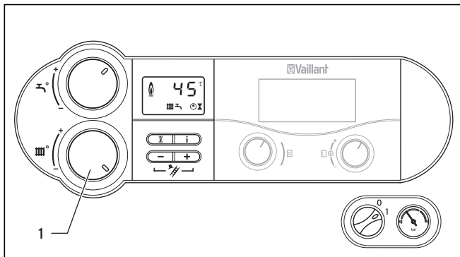
Abb. 5.12 Vorlauftemperatur einstellen mit Regelgerät
