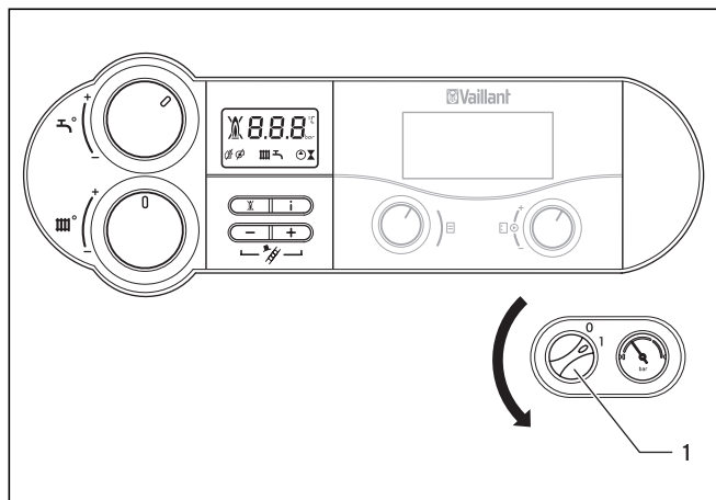
Abb. 5.16 Gerät ausschalten
