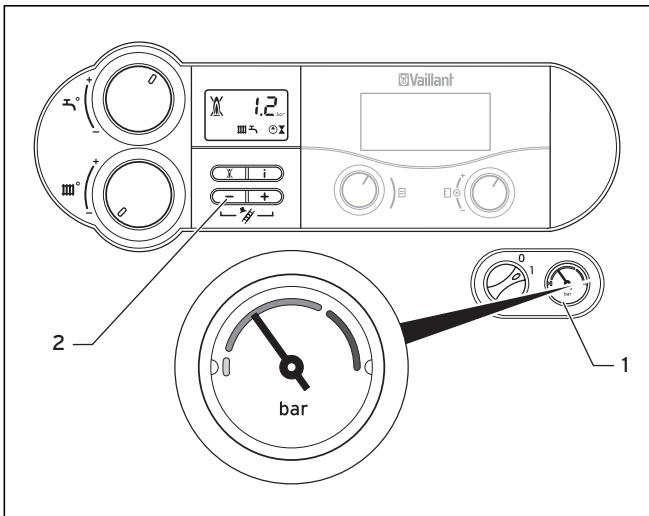
Abb. 5.15 Heizungsanlage füllen
