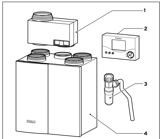
3.2 Wohnraumlüftungsgerät recoVAIR
