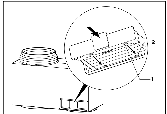
7.5 Bypass-Filter zurückschieben
