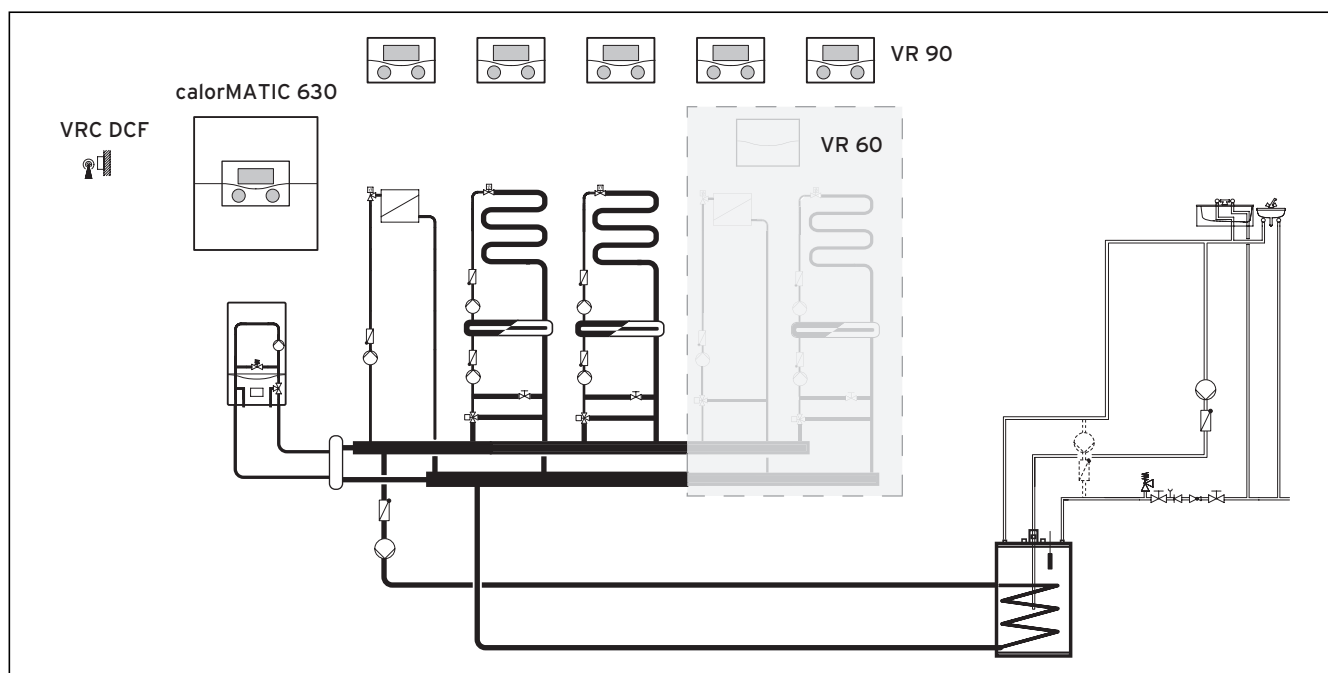
Abb. 3.1 Systemübersicht
