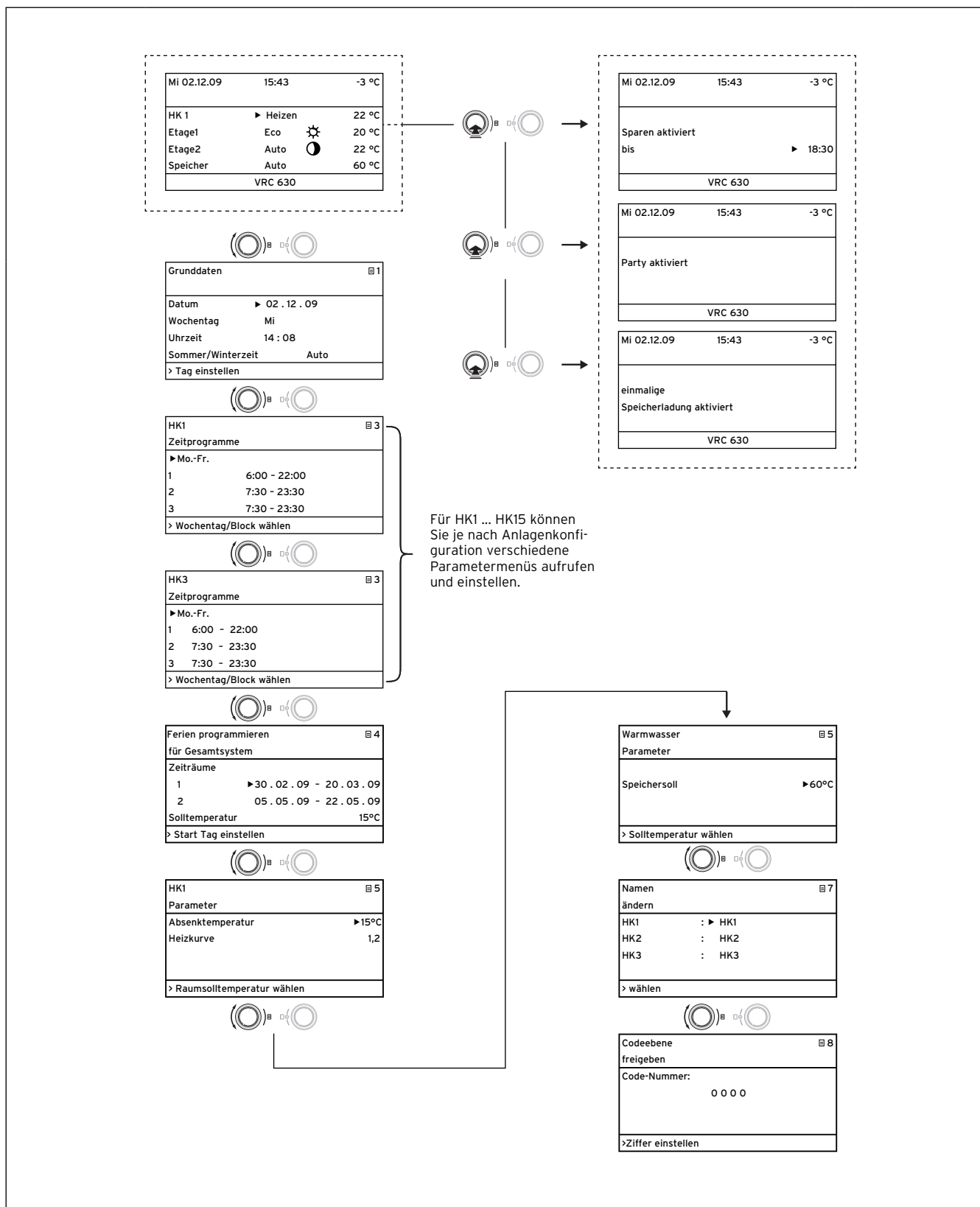
Abb. 3.6 Menüstruktur Betreiberebene
