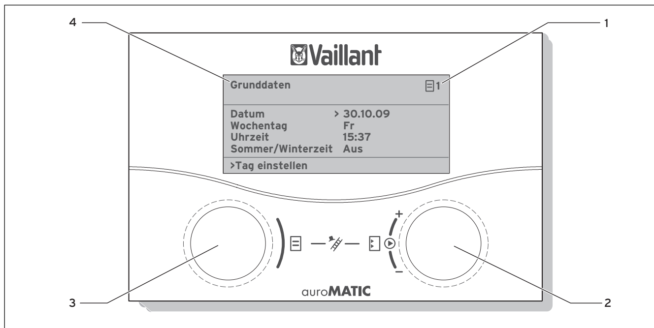
Abb. 3.5 Übersicht Bedienelemente
