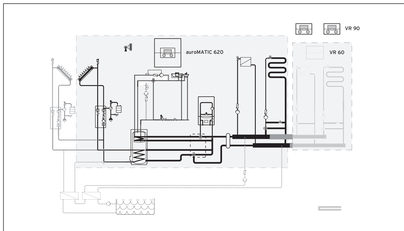
Abb. 3.1 Systemübersicht
