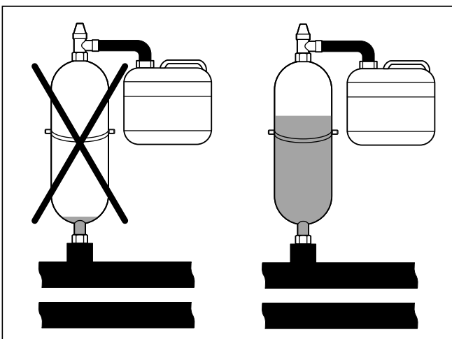
6.1 Füllstand des Sole-Ausgleichsbehälters
