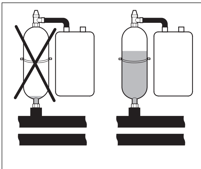
Abb. 6.1 Füllstand des Sole-Ausgleichsbehälters
