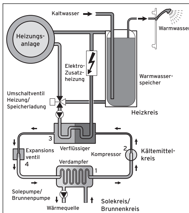
Abb. 3.3 Funktionsweise der Wärmepumpe
