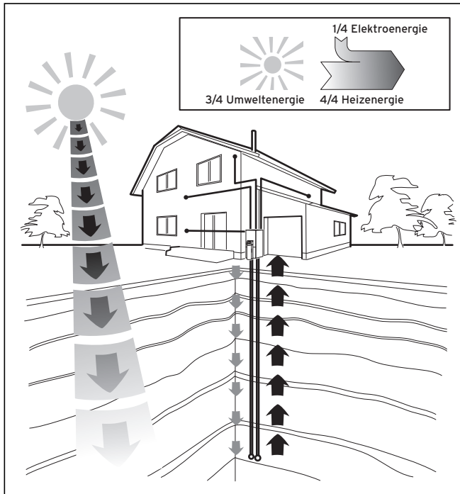
Abb. 3.1 Nutzung der Wärmequelle Erdwärme
