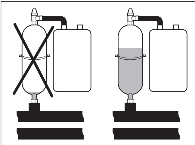
Abb. 6.1 Füllstand des Sole-Ausgleichsbehälters
