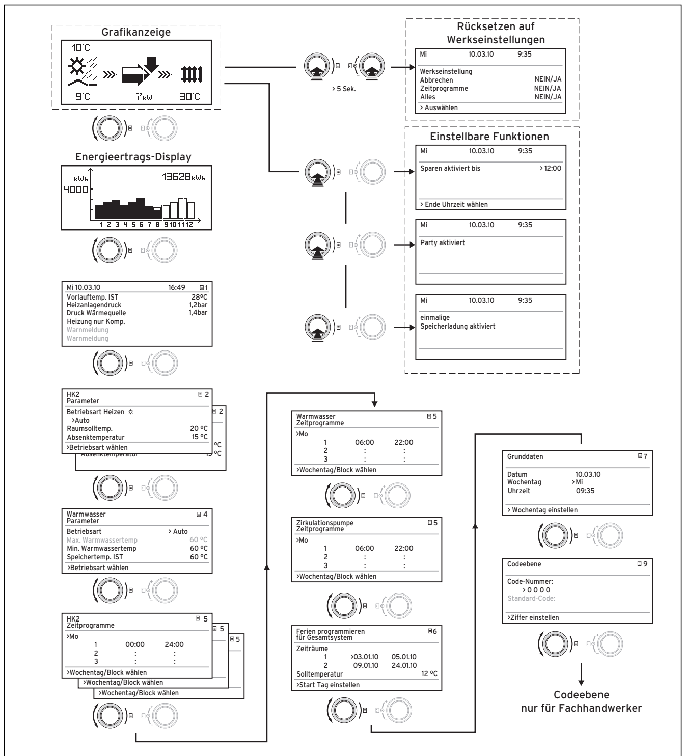
Abb. 4.2 Menüabfolge in der Betreiberebene
