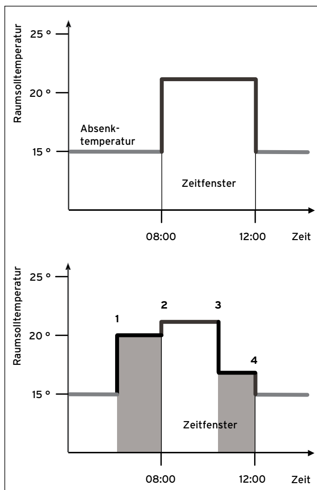
Abb. 4.2 Gültigkeitsdauer von Sollwert-Änderungen (hier: Raumsolltemperatur)
