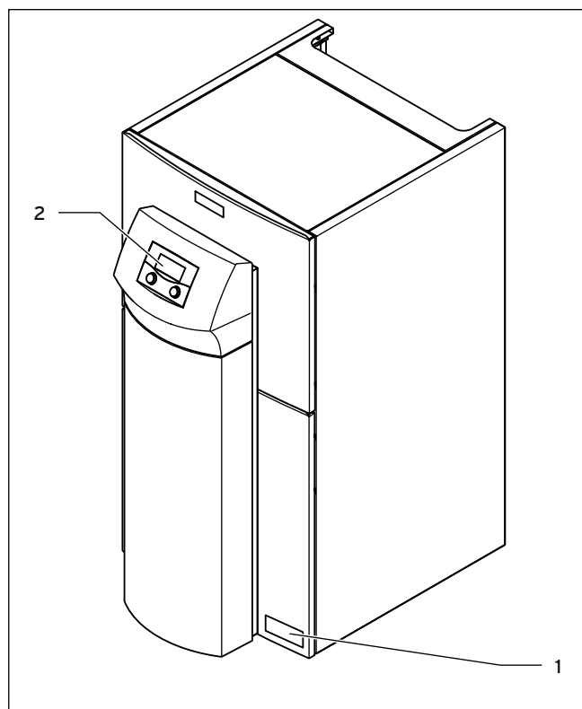
Abb. 3.1 Vorderansicht Inneneinheit
