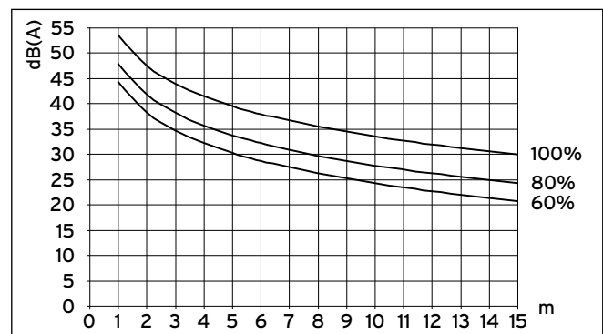
Abb. 6.2 Schalldruckpegel einer Außeneinheit in dB(A) in Abhängigkeit von der Entfernung und der Lüfterdrehzahl für VWL 81/3 S bei Freifeldaufstellung
