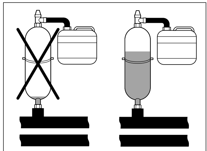
Abb. 6.6 Füllstand des Sole-Ausgleichsbehälters
