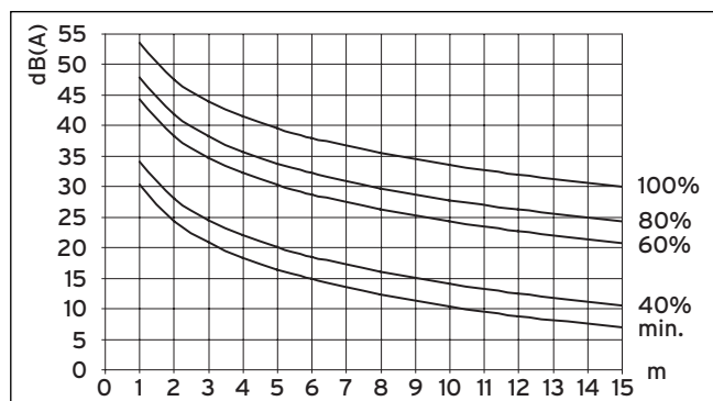
Abb. 6.2 Schalldruckpegel einer Außeneinheit in dB(A) in Abhängigkeit von der Entfernung und der Lüfterdrehzahl für VWL 81/3 S bei Freifeldaufstellung
