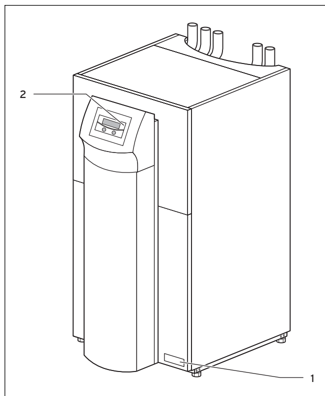
Abb. 3.1 Vorderansicht Inneneinheit
