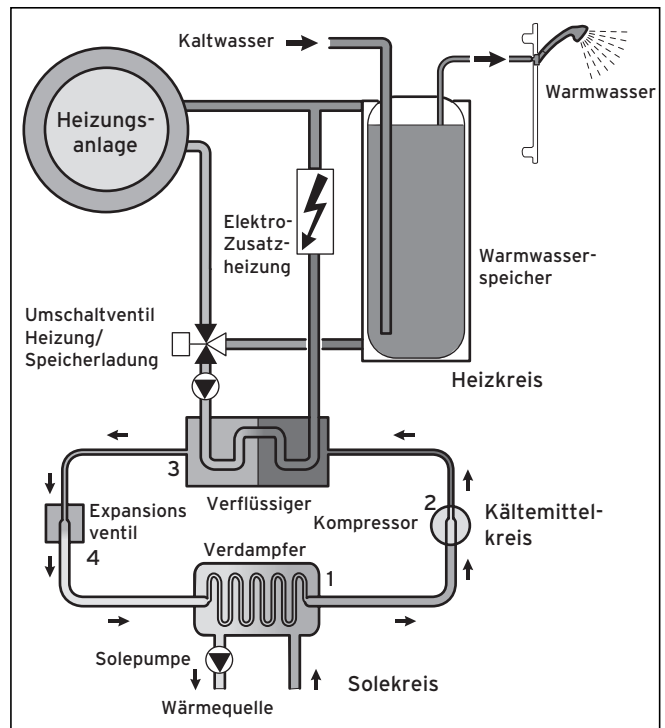
Abb. 3.4 Funktionsweise der Wärmepumpe (Inneneinheit)
