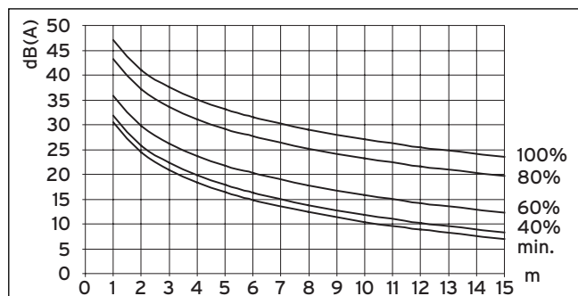
Abb. 6.1 Schalldruckpegel einer Außeneinheit in dB(A) in Abhängigkeit von der Entfernung und der Lüfterdrehzahl für VWL 61/3 S bei Freifeldaufstellung
