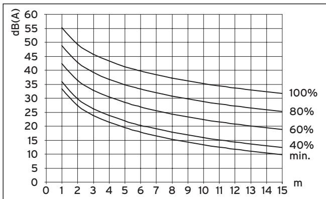
Abb. 6.4 Schalldruckpegel zweier Außeneinheiten in dB(A) in Abhängigkeit von der Entfernung und der Lüfterdrehzahl für VWL 141/3 S bei Freifeldaufstellung
