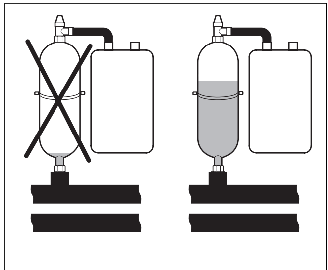
Abb. 6.6 Füllstand des Sole-Ausgleichsbehälters
