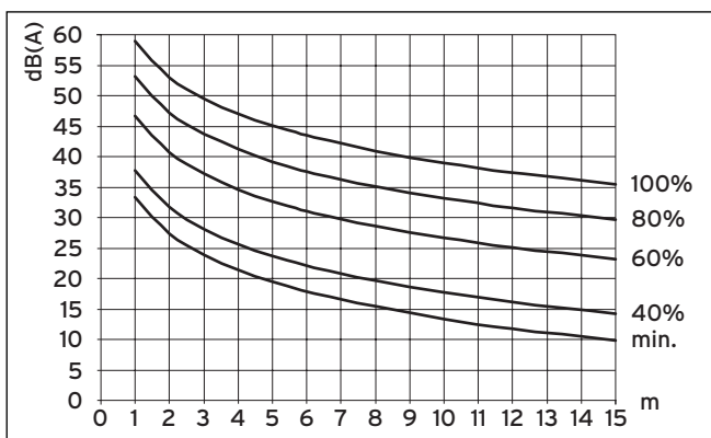
Abb. 6.5 Schalldruckpegel zweier Außeneinheiten in dB(A) in Abhängigkeit von der Entfernung und der Lüfterdrehzahl für VWL 171/3 S bei Freifeldaufstellung
