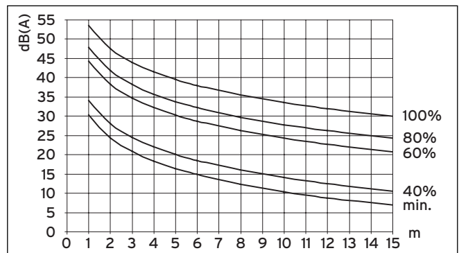
Abb. 3.2 Schalldruckpegel einer Außeneinheit in dB(A) in Abhängigkeit von der Entfernung und der Lüfterdrehzahl für VWL 81/3 S bei Freifeldaufstellung
