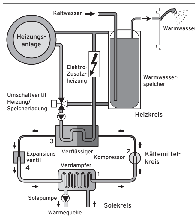
Abb. 3.7 Funktionsweise der Wärmepumpe (Inneneinheit)
