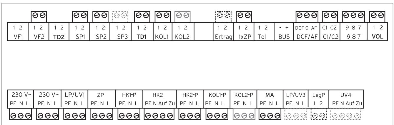
Abb. 4.20 Benötigte ProE-Steckplätze
