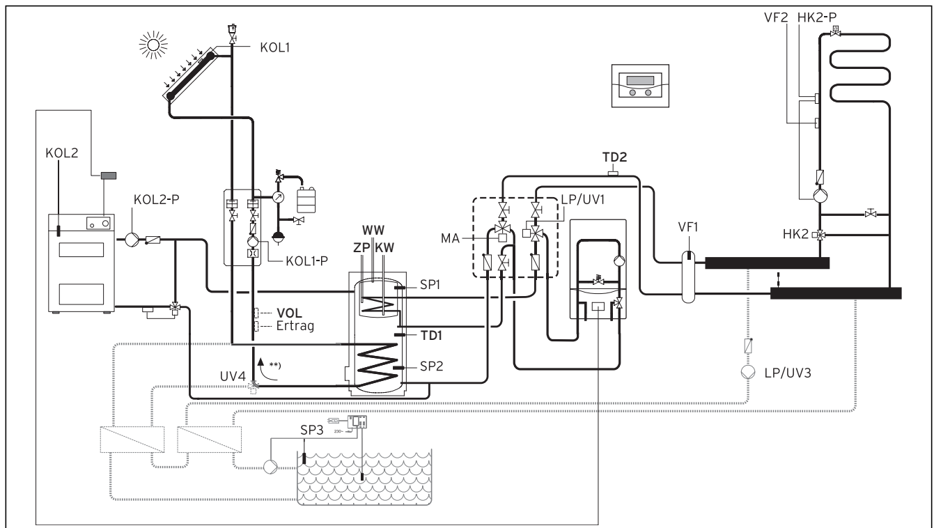
Abb. 4.5 Hydraulikplan 2
