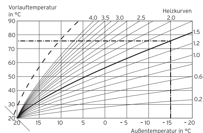
Abb. Heizkurve
