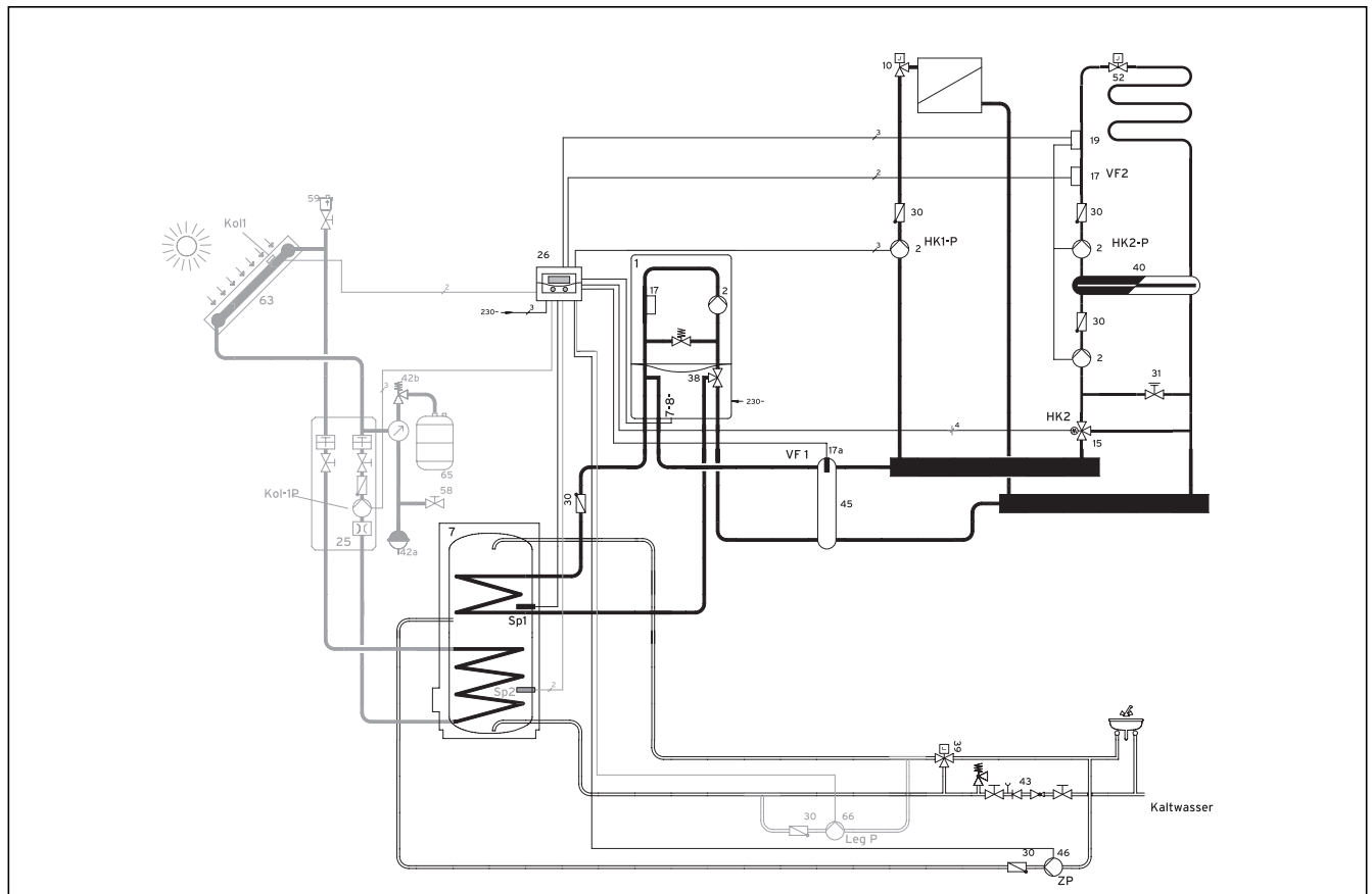
Abb. 4.13 Hydraulikplan 3.3
