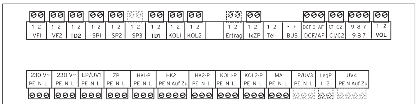
Abb. 4.6 Benötigte ProE-Steckplätze
