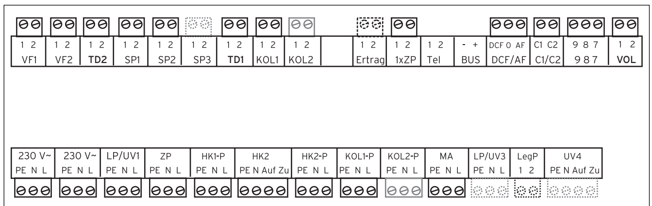
Abb. 4.14 Benötigte ProE-Steckplätze
