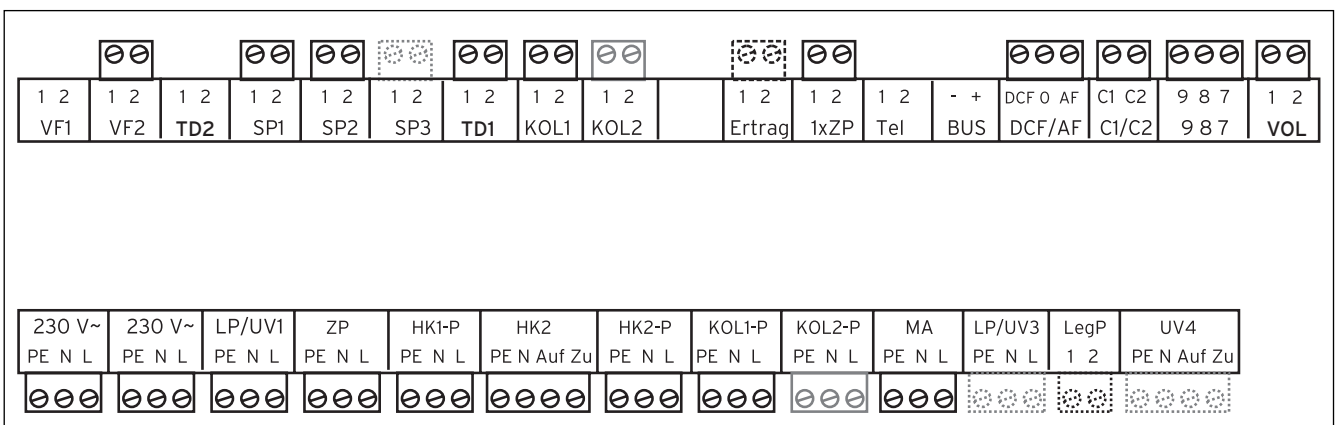
Abb. 4.24 Benötigte ProE-Steckplätze
