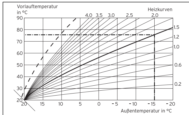
Abb. Heizkurve
