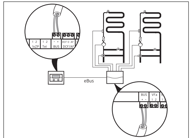
Abb. 4.33 Weitere Mischerkreise
