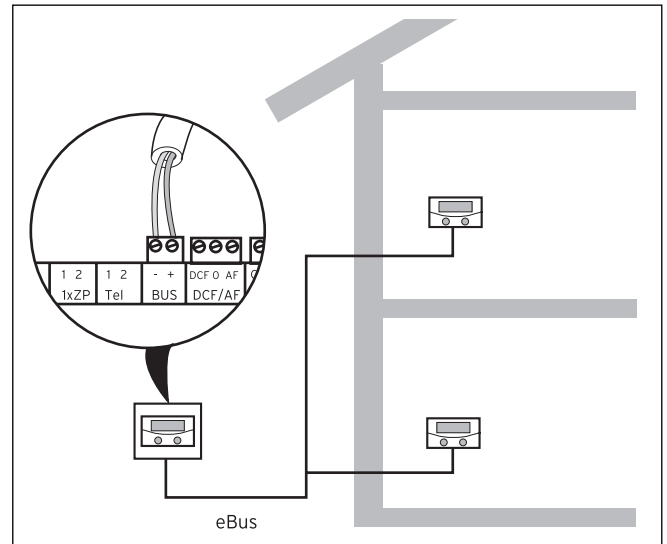
Abb. 4.32 Fernbediengeräte anschließen
