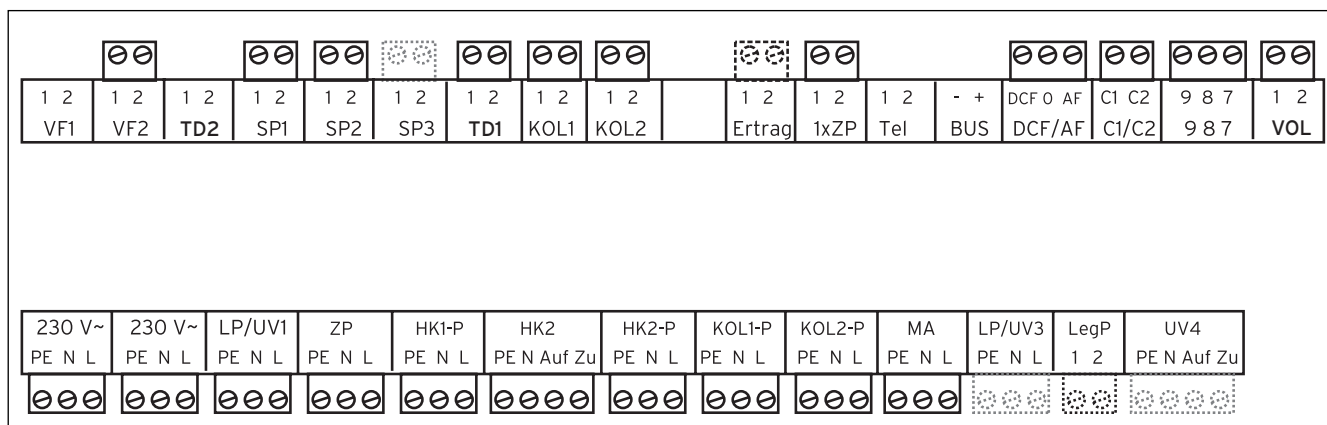
Abb. 4.22 Benötigte ProE-Steckplätze
