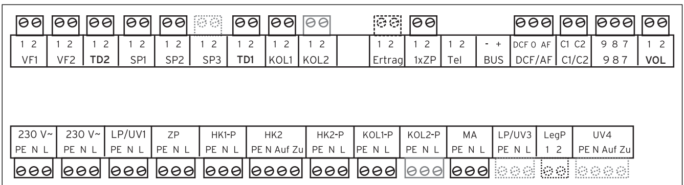
Abb. 4.12 Benötigte ProE-Steckplätze
