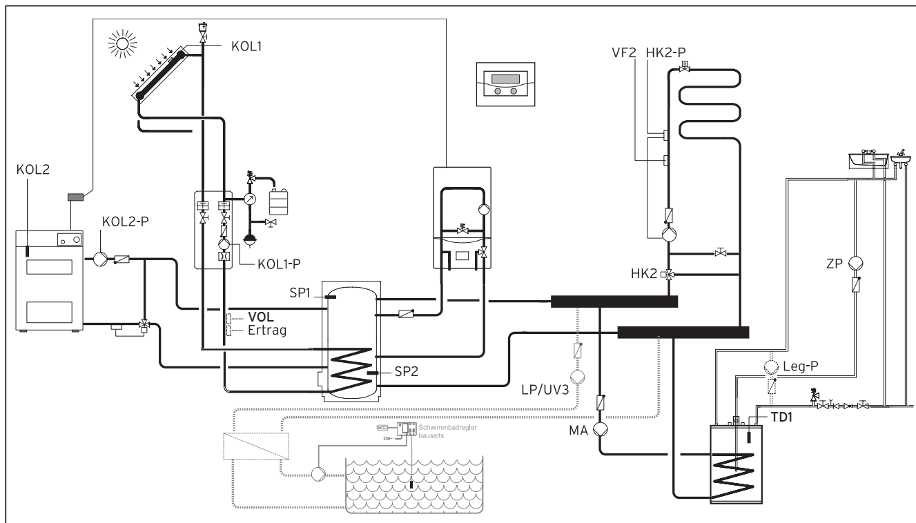
Abb. 4.21 Hydraulikplan 6
