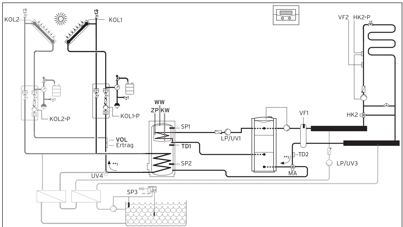
Abb. 4.7 Hydraulikplan 3
