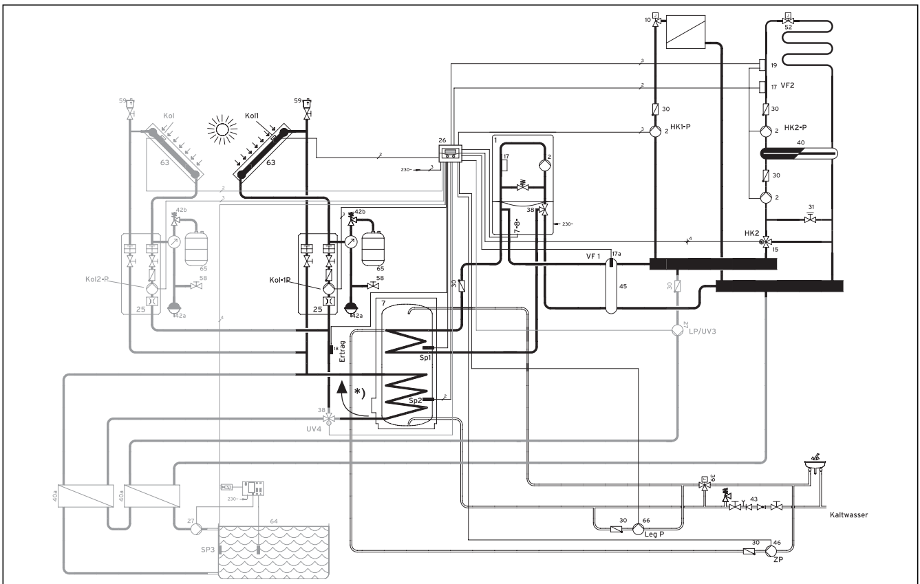
Abb. 4.11 Hydraulikplan 3.2
