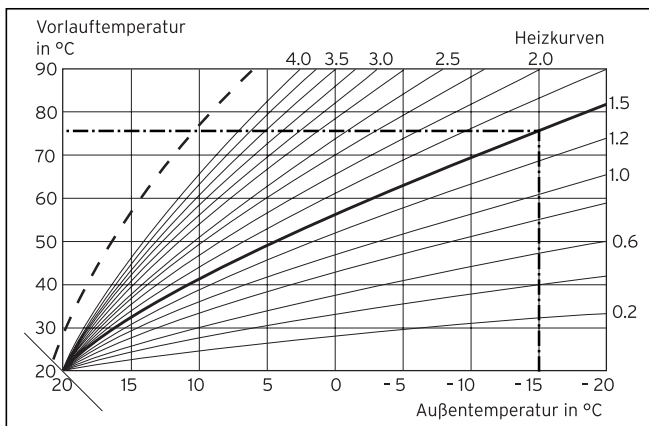
Abb. 6.21 Heizkurve
