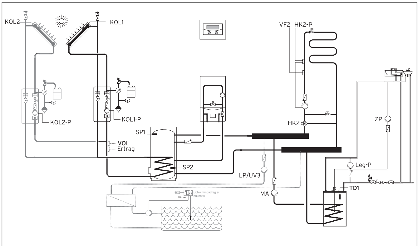
Abb. 4.19 Hydraulikplan 5
