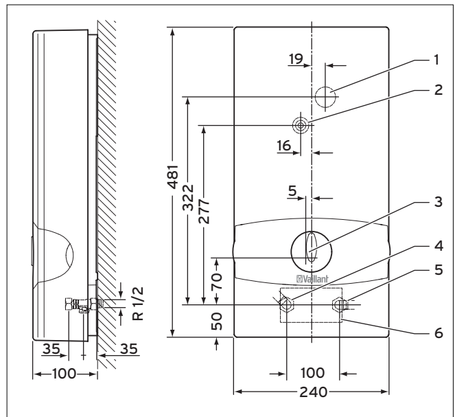
Abb. 4.3 Geräteabmessungen
