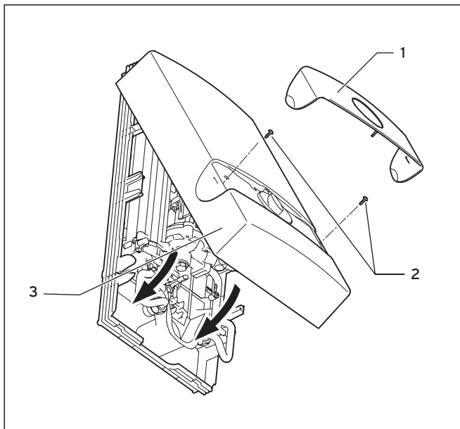
Abb. 5.2 Geräteverkleidung anbringen
