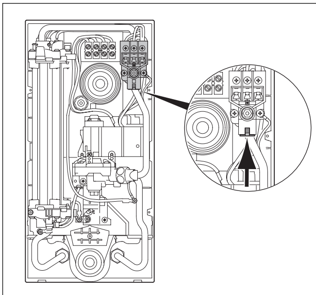
Abb. 5.1 Sicherheitsschalter
