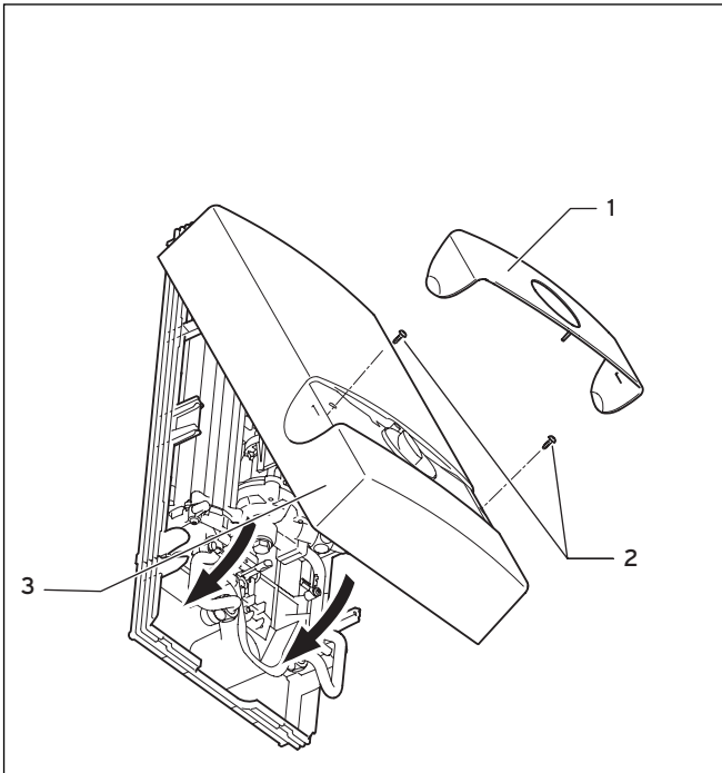
Abb. 5.2 Geräteverkleidung anbringen
