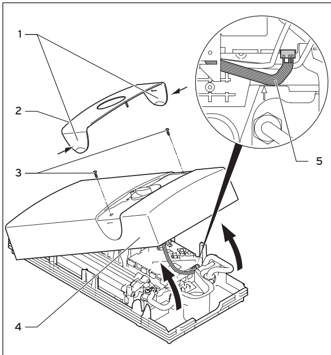
Abb. 4.5 Geräteverkleidung abnehmen
