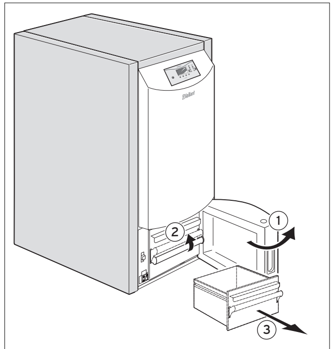
Abb. 4.6 Zweiteilige Aschebehälter herausziehen
