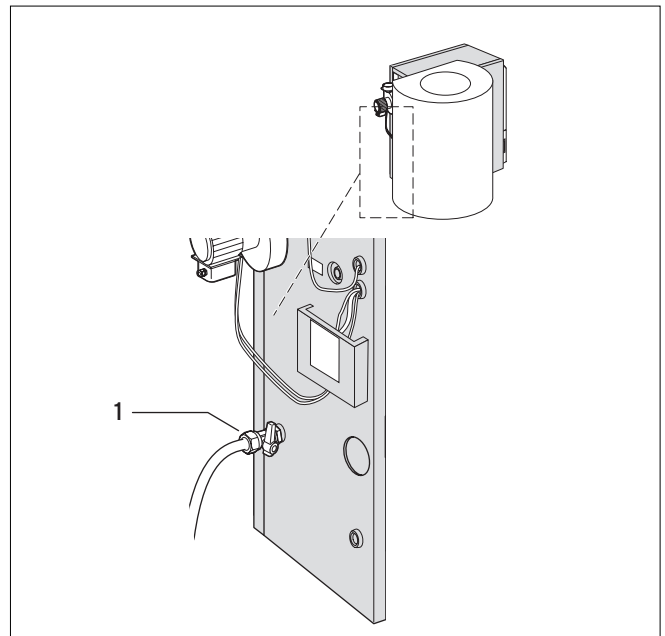
Abb. 4.10 Heizungsanlage füllen
