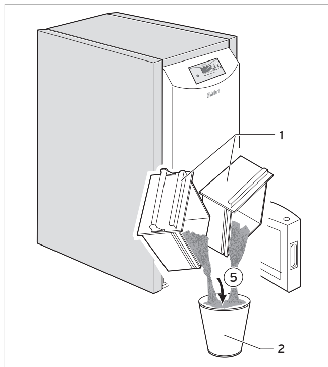
Abb. 4.8 Aschebehälter leeren
