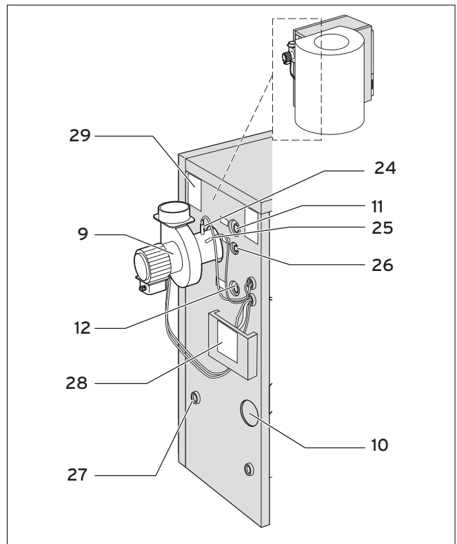
Abb. 3.2 Rückansicht des Pellet-Heizkessels mit Saugaustragung
