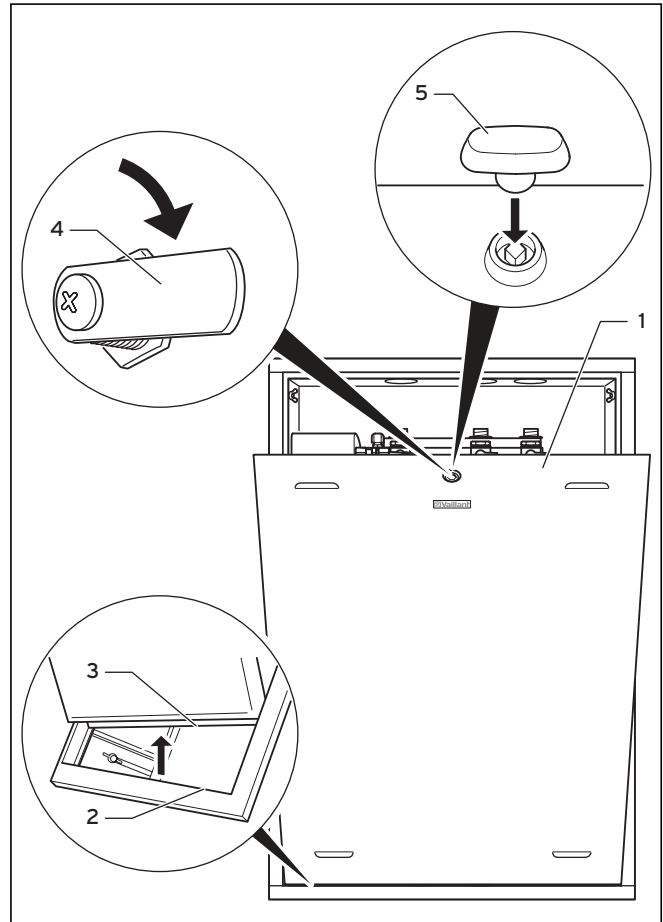
Abb. 4.1 Öffnen der Verkleidungstür
