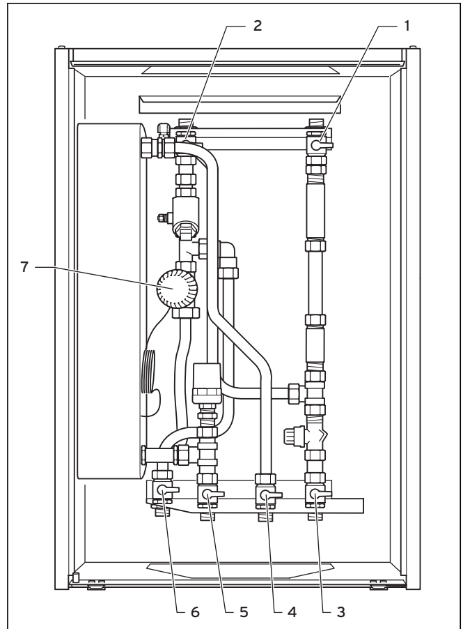
Abb. 5.2 Bedienelemente VSW 15-35 (Auslieferungszustand)
