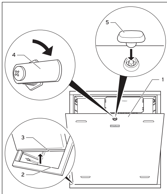
Fig. 5.1 Apertura dello sportello del rivestimento
