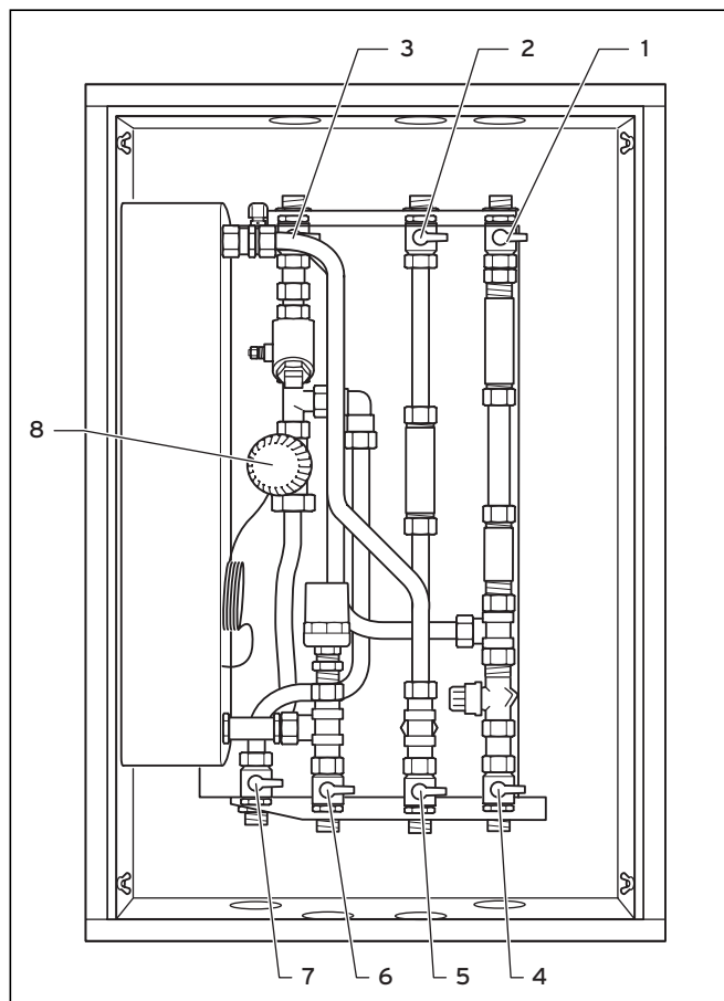
Fig. 4.2 Elementi di comando (stato al momento della consegna)
