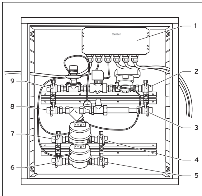
Fig. 5.2 Elementi di comando VS 15 I (stato al momento della consegna)
