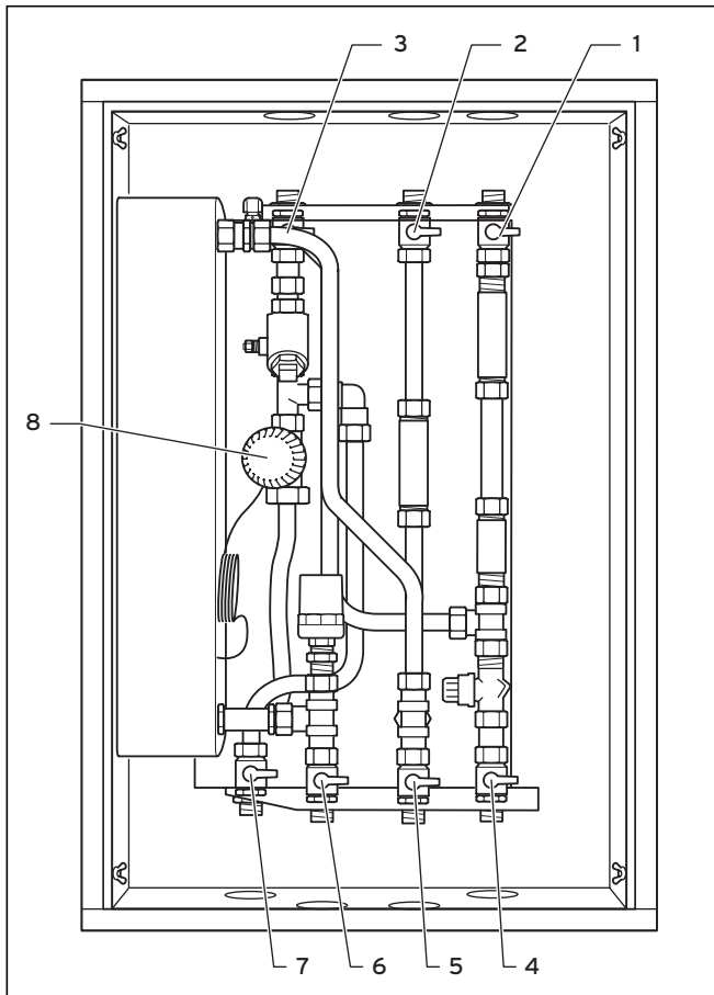
Abb. 4.2 Bedienelemente (Auslieferungszustand)
