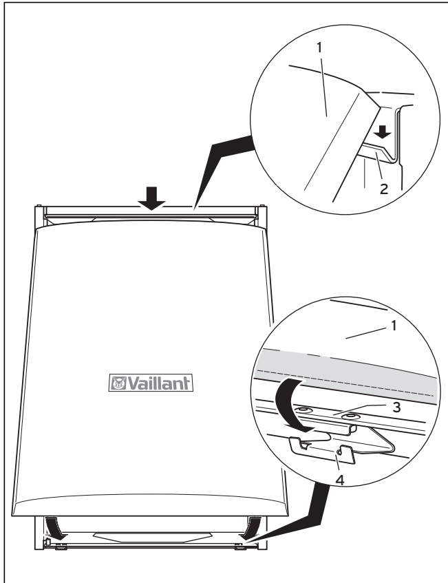
Abb. 5.1 Öffnen der Verkleidungstür
