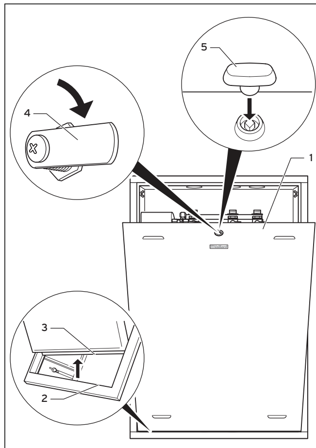
Fig. 4.1 Apertura dello sportello del rivestimento
