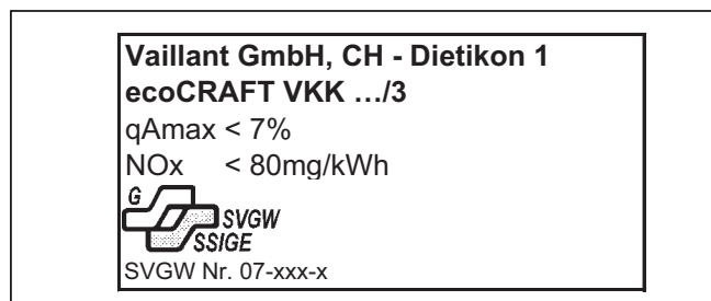
Abb. 1.2 Zusatz-Typenschild Schweiz
