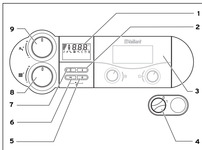
Fig. 4.1 Elementi di comando ecoCRAFT exclusiv
