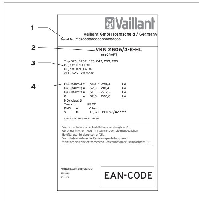
Abb. 1.1 Typenschild
