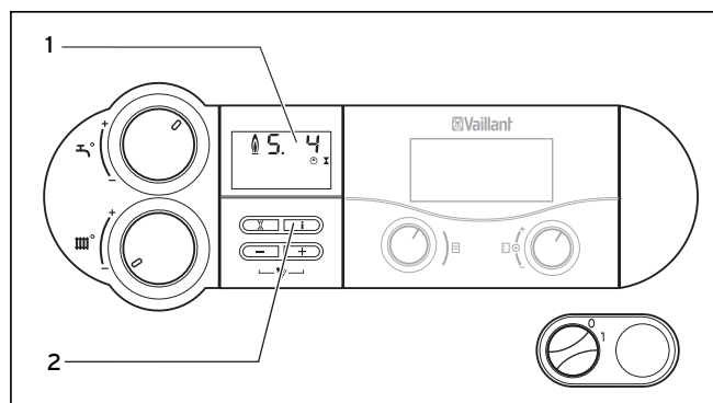
Abb. 4.10 Statusanzeigen
