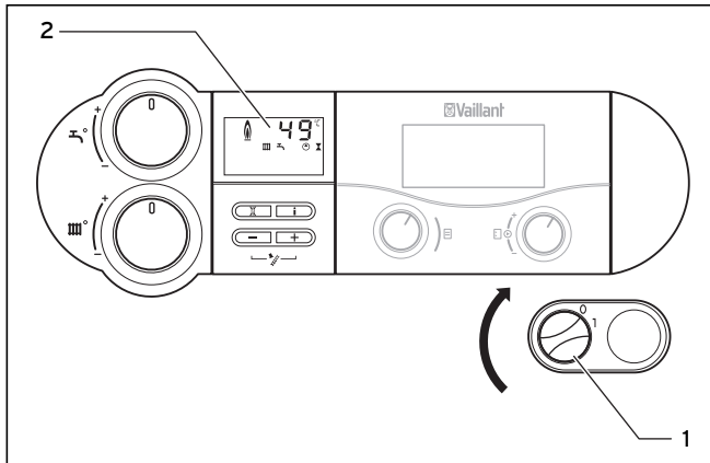
Abb. 4.4 Gerät einschalten
