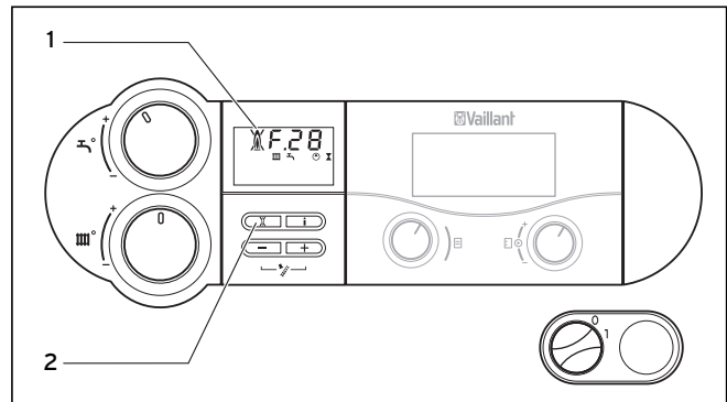
Abb. 4.11 Entstörung
