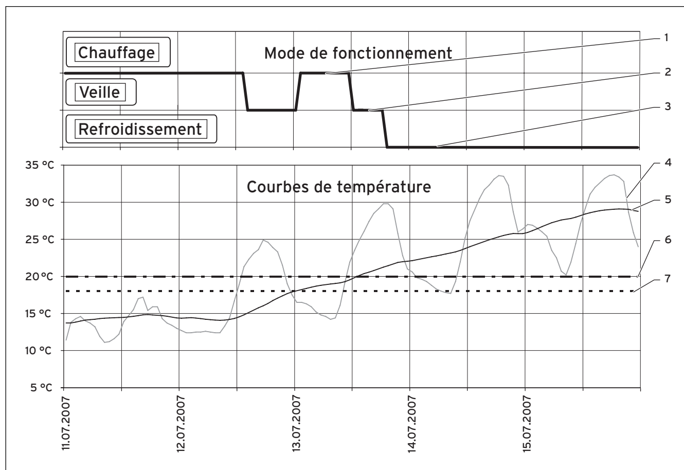
Fig. 3.5 Exemple d'un passage dépendant de la température extérieure entre le mode de chauffage et celui de refroidissement
