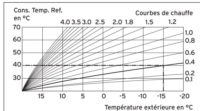
Fig. 10.1 Diagramme des courbes de chauffage
