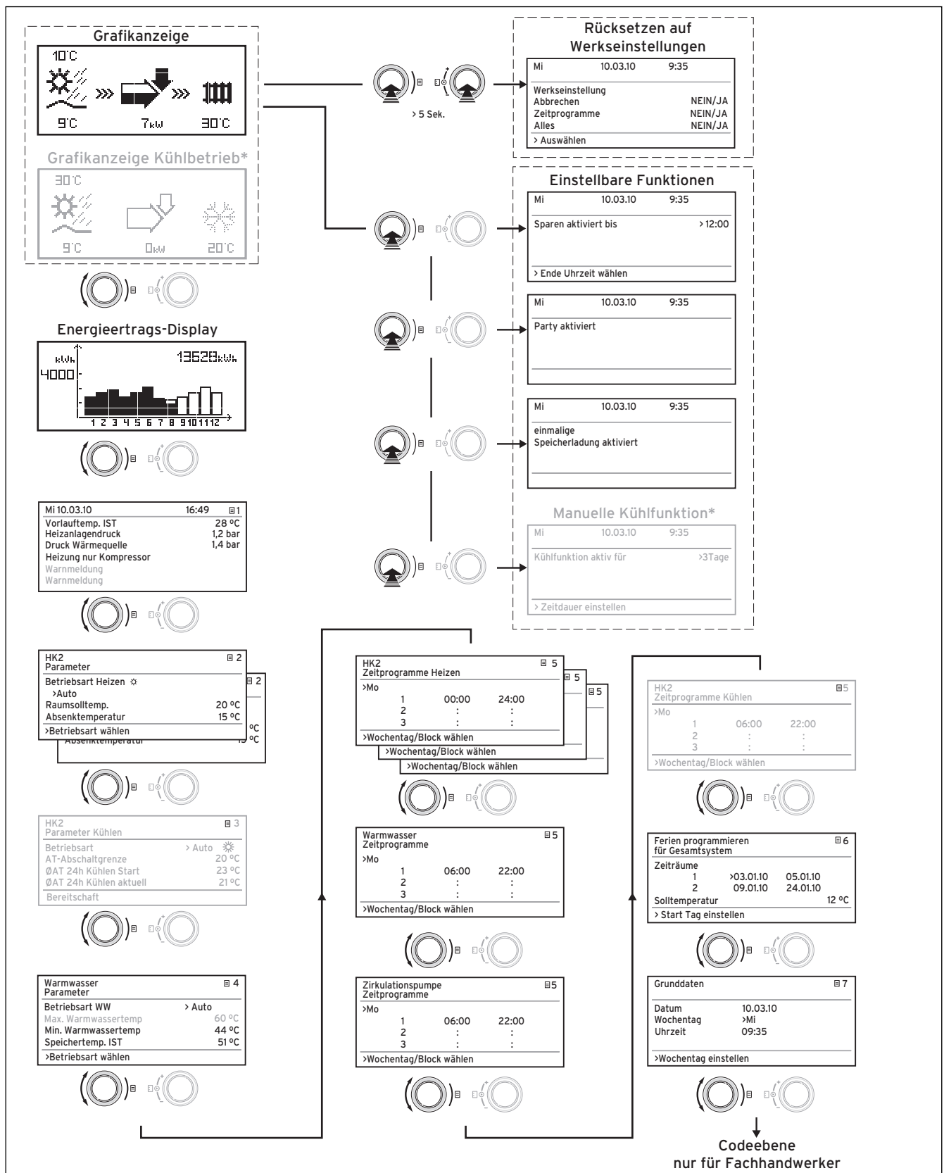
Abb. 4.2 Menüabfolge
