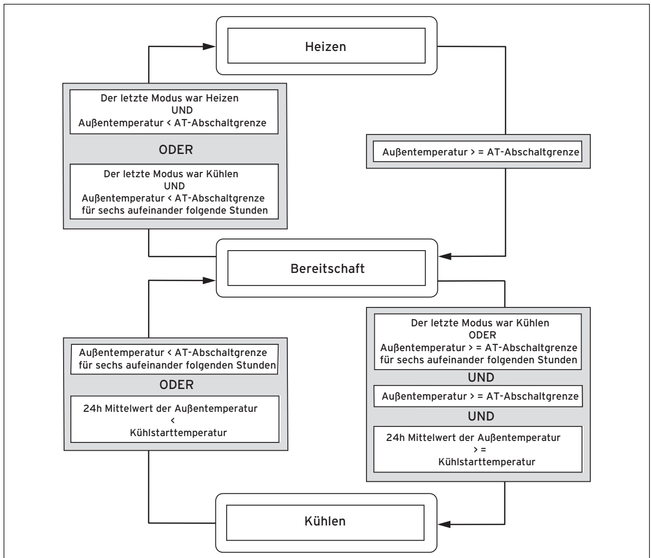
Abb. 3.4 Übergangsschema
