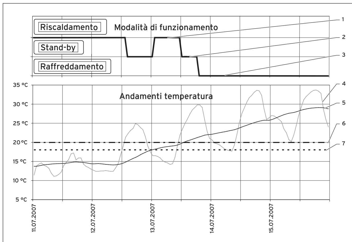
Fig. 3.5 Esempio di transizione, dovuta alla temperatura esterna, tra riscaldamento e raffreddamento
