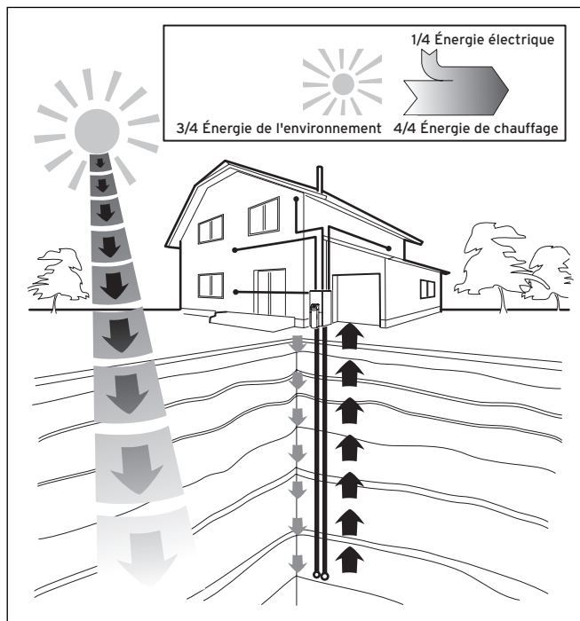
Fig. 3.2 Exploitation de la source géothermique
