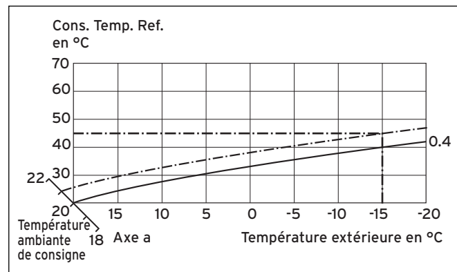
Fig. 10.2 Déplacement parallèle de la courbe de chauffage
