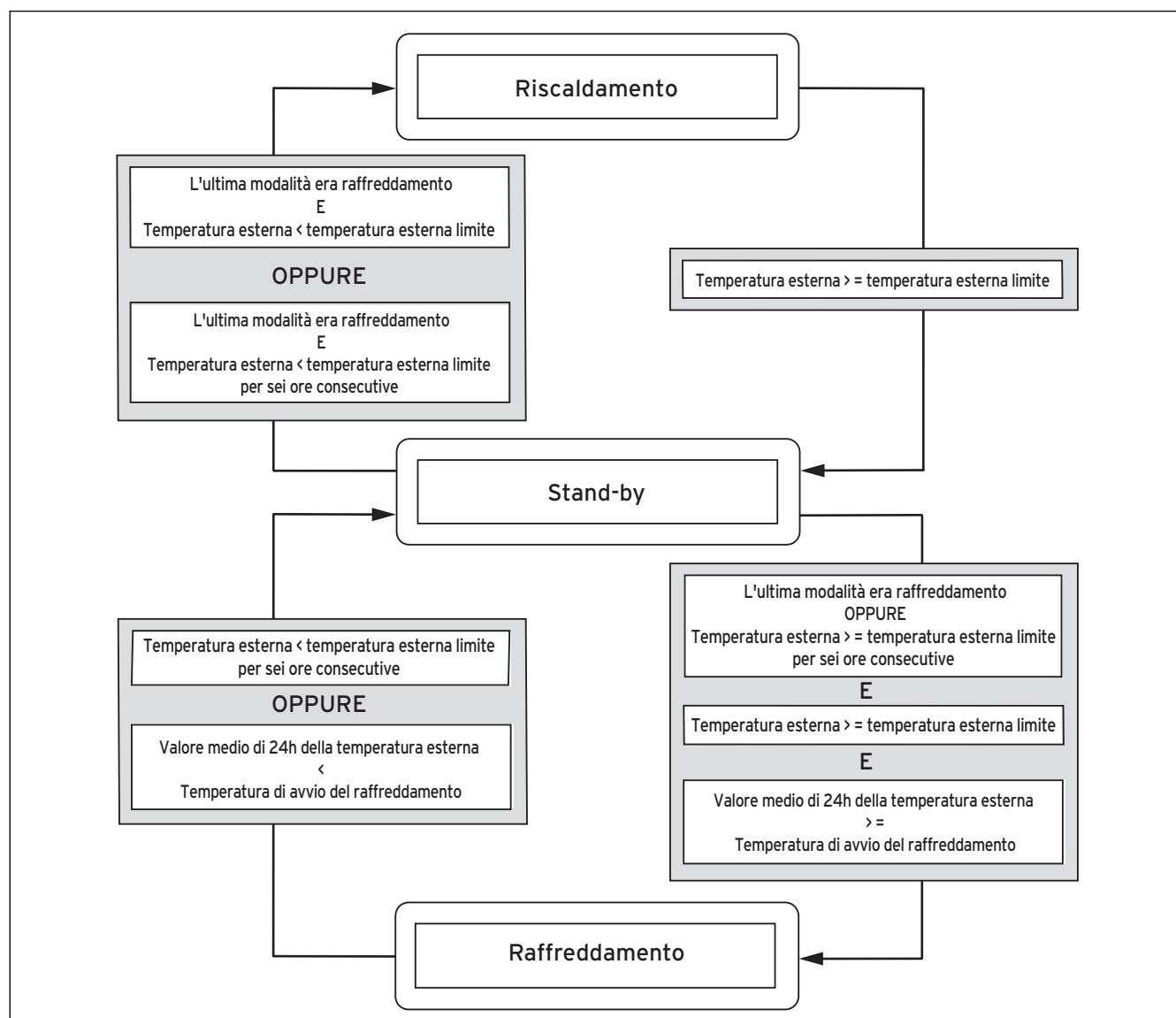
Fig. 3.4 Schema di transizione
