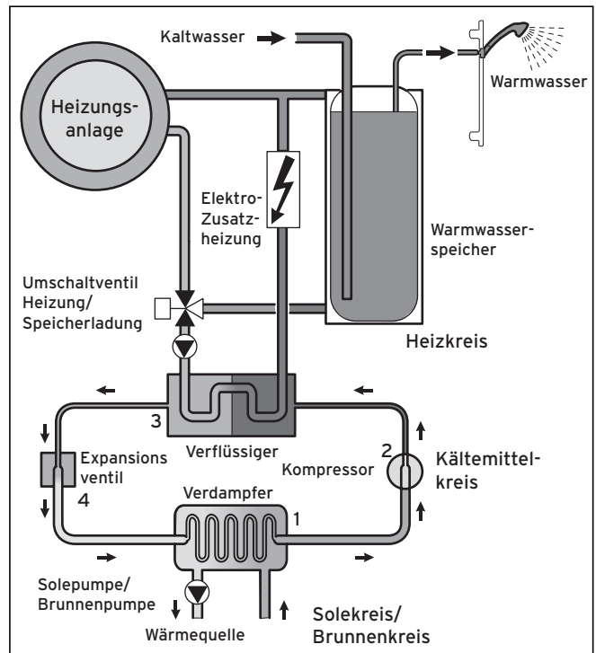
Abb. 3.3 Funktionsweise der Wärmepumpe
