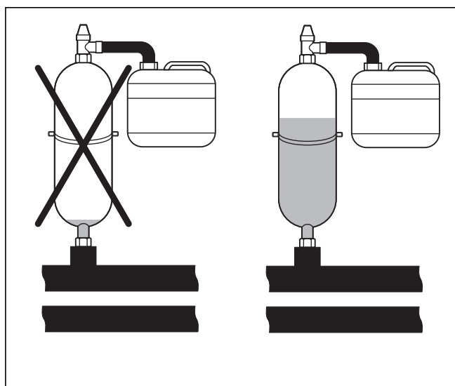
Fig. 6.1 Livello del serbatoio di compensazione della miscela incongela- bile
