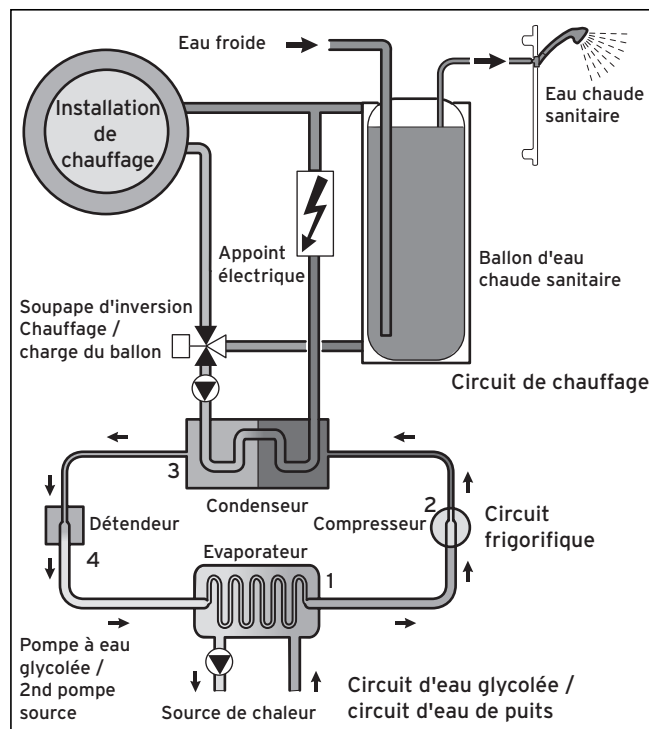
Fig. 3.3 Fonctionnement de la pompe à chaleur
