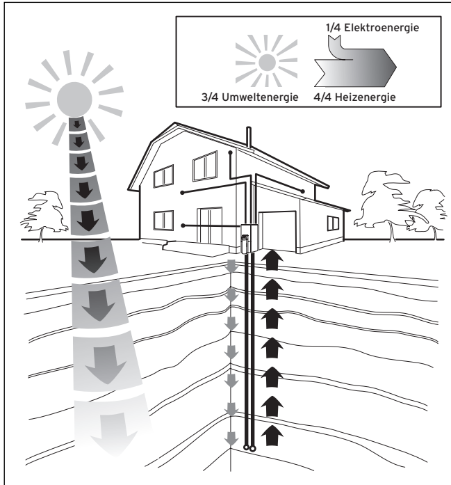
Abb. 3.2 Nutzung der Wärmequelle Erdwärme
