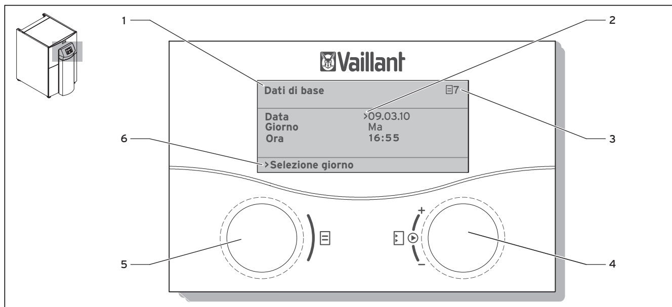
Fig. 4.1 Superficie di comando della centralina
