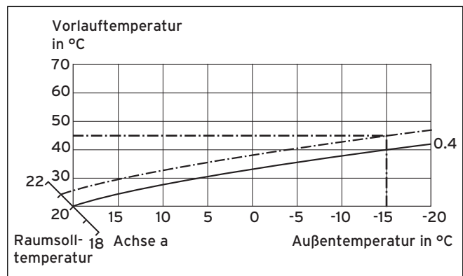
Abb. 10.2 Parallelverschiebung der Heizkurve
