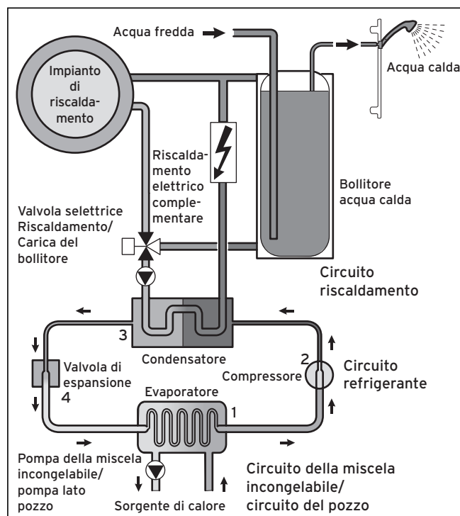
Fig. 3.3 Modalità di funzionamento della pompa di calore
