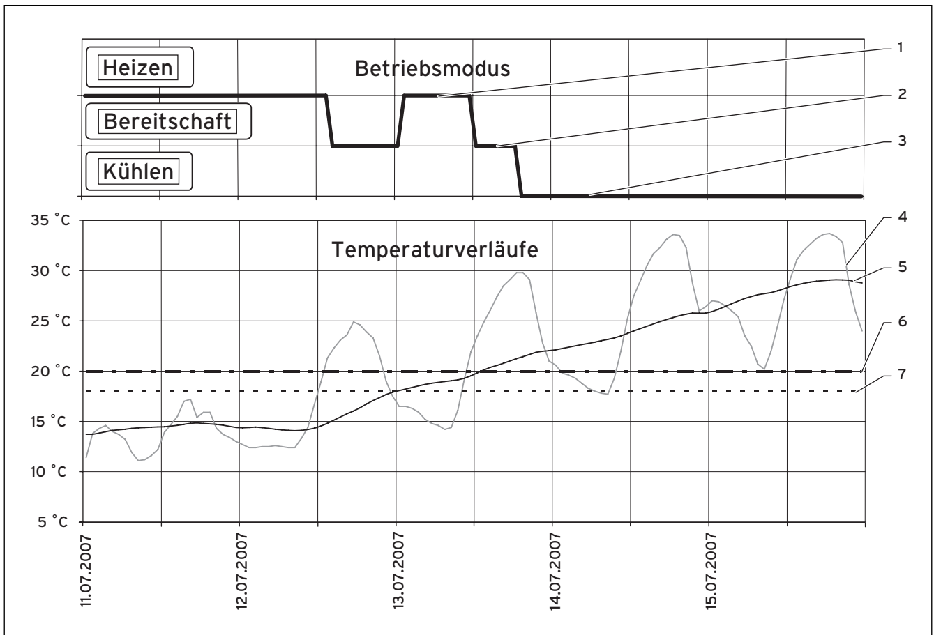
Abb. 3.5 Beispiel für eine außentemperaturabhängige Umschaltung zwischen Heizen und Kühlen
