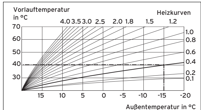
Abb. 10.1 Diagramm Heizkurven
