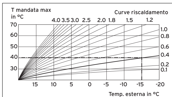
Fig. 10.1 Grafico con curve di riscaldamento
