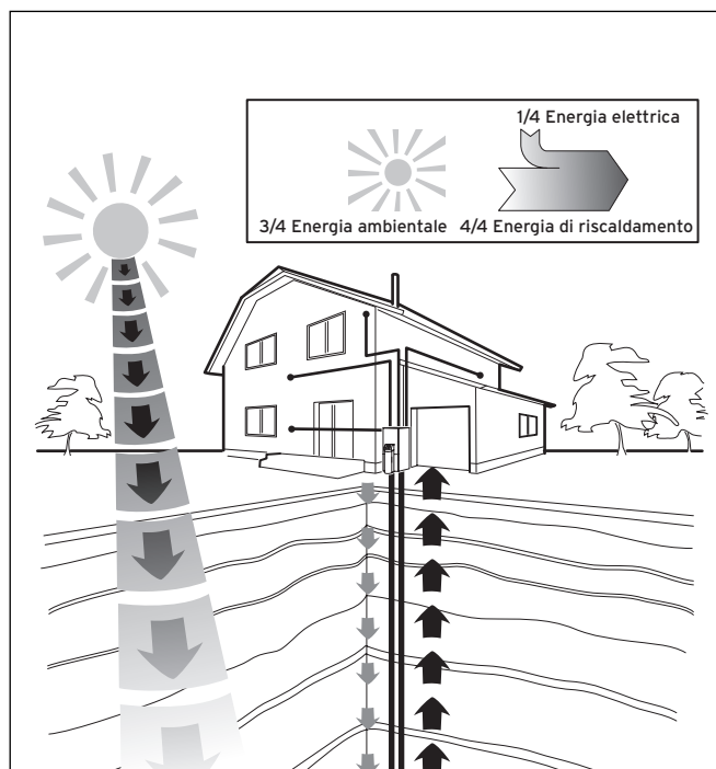
Fig. 3.2 Sfruttamento del calore geotermico come sorgente di calore
