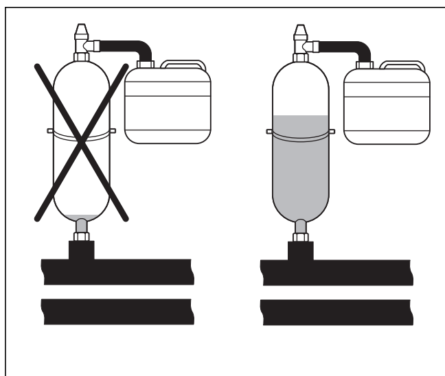
Fig. 6.1 Niveau d'eau glycolée dans le réservoir de compensation
