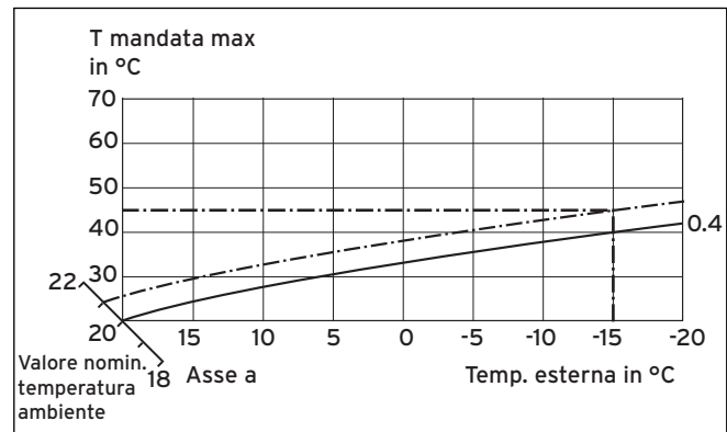
Fig. 10.2 Spostamento in parallelo della curva di riscaldamento
