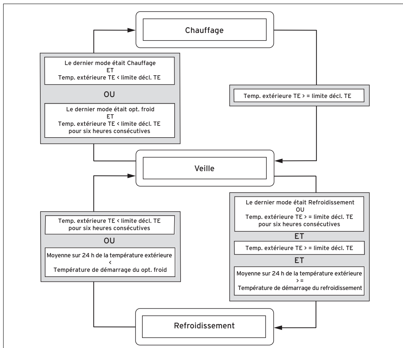
Fig. 3.4 Schéma de transition
