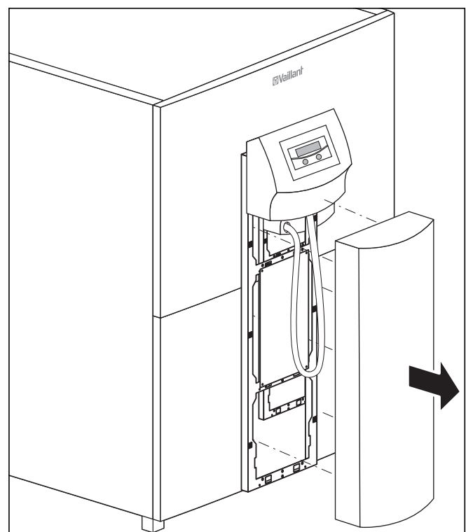
Abb. 1.1 Säulenabdeckung entfernen
