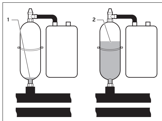
Fig. 5.6 Niveau d'eau glycolée du réservoir de compensation
