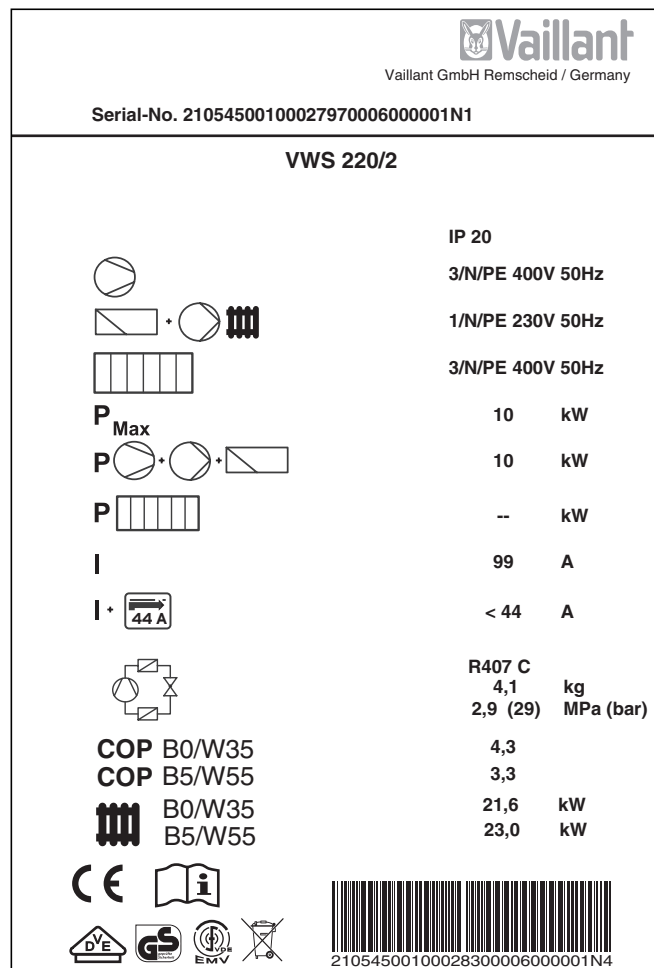
Fig. 7.1 Exemple de plaque signalétique
