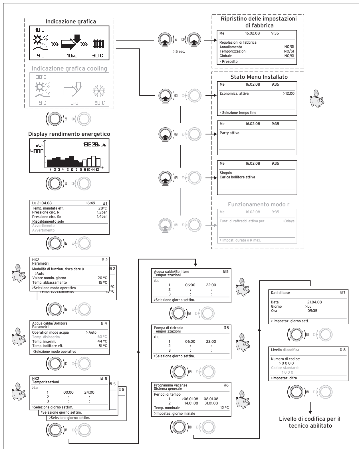
Fig. 5.2 Schermate del livello utente
