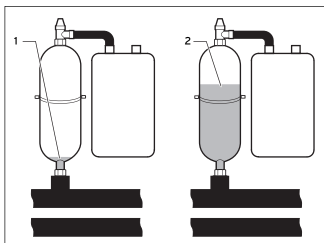
Fig. 5.6 Livello del serbatoio di compensazione miscela incongela- bile
