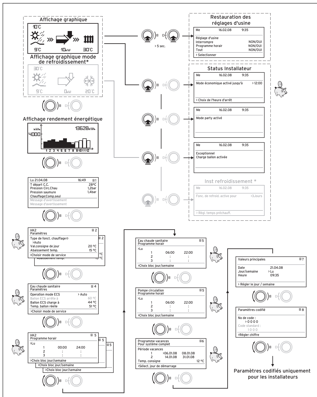
Fig. 5.2 Ecrans du niveau de l'utilisateur
