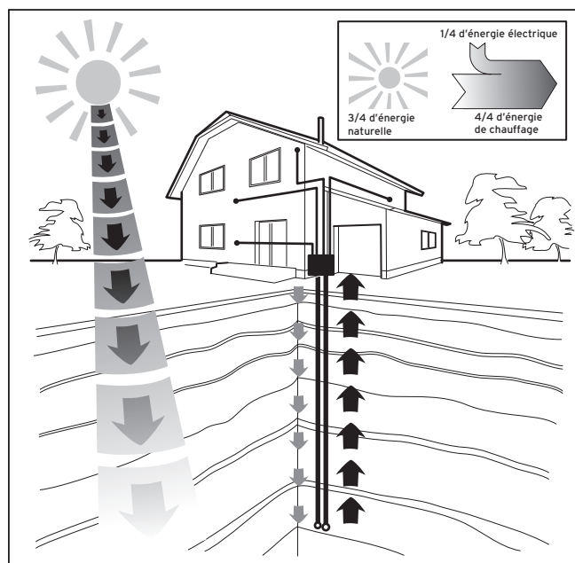
Fig. 3.1 Utilisation de la géothermie ou de la nappe phréatique
