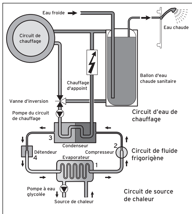
Fig. 3.2 Fonctionnement de la pompe à chaleur
