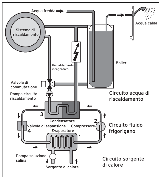
Fig. 3.2 Modalità di funzionamento della pompa di calore
