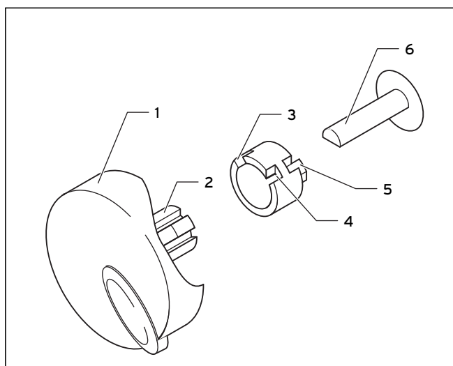
Fig. 9.1 Délimitation de la plage de réglage de la température
