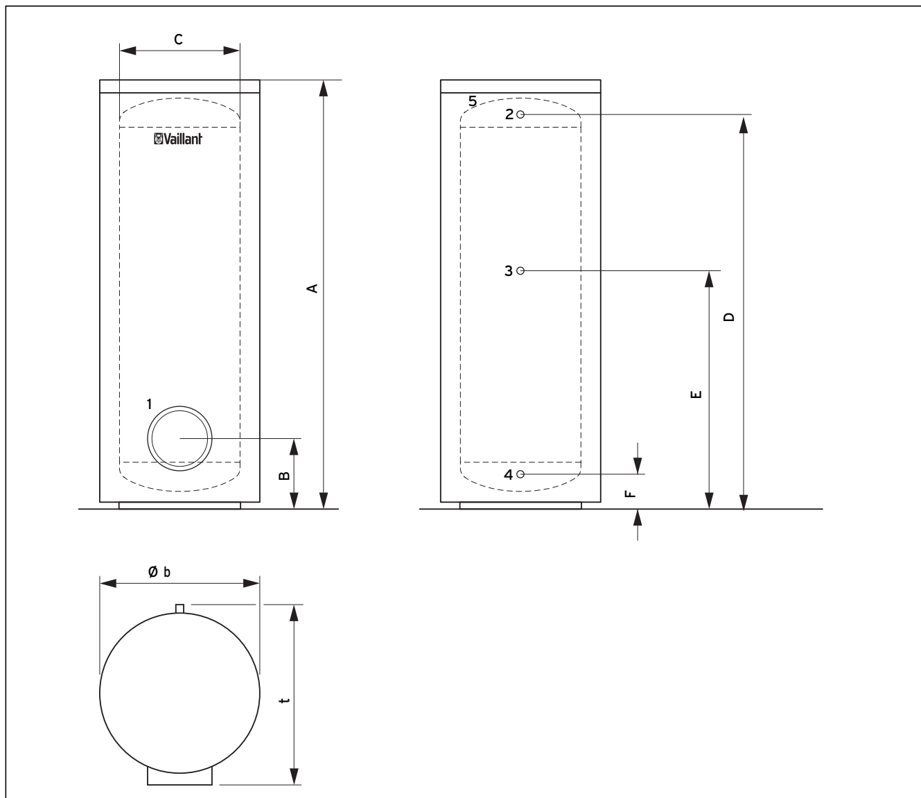
Fig. 7.2 Dimensioni
