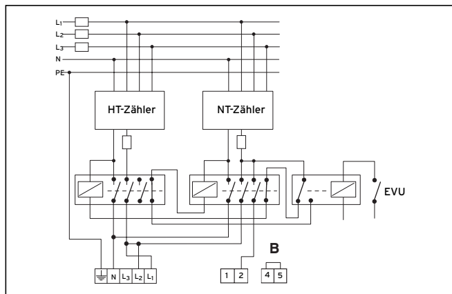
Abb. 8.2 Anschluss einphasig
