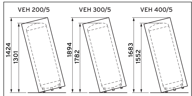
Fig. 7.1 Cote de basculement
