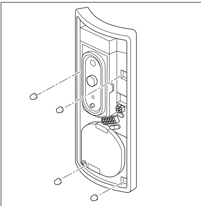
Fig. 7.15 Démontage de l'E-Box
