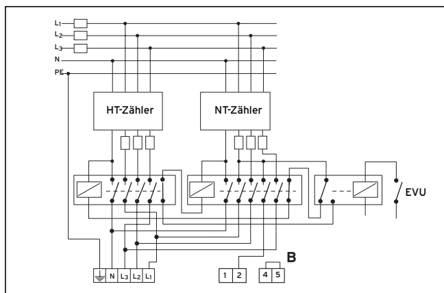
Abb. 8.4 Anschluss dreiphasig
