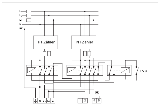
Abb. 8.3 Anschluss zweiphasig
