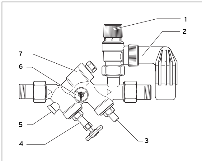
Fig. 7.19 Installation des groupes de sécurité
