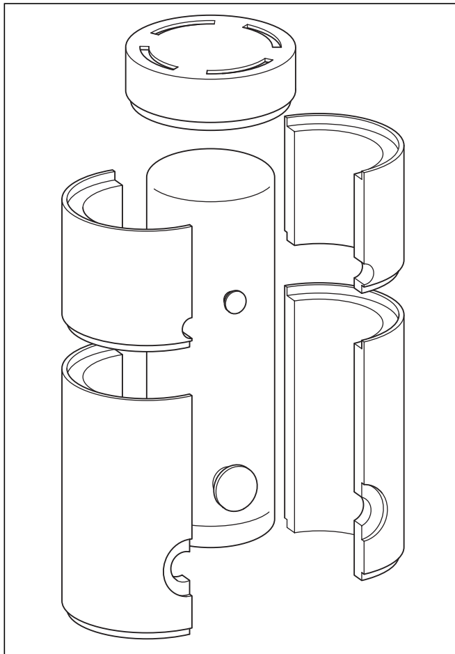
7.18 Rimozione dell'isolamento
