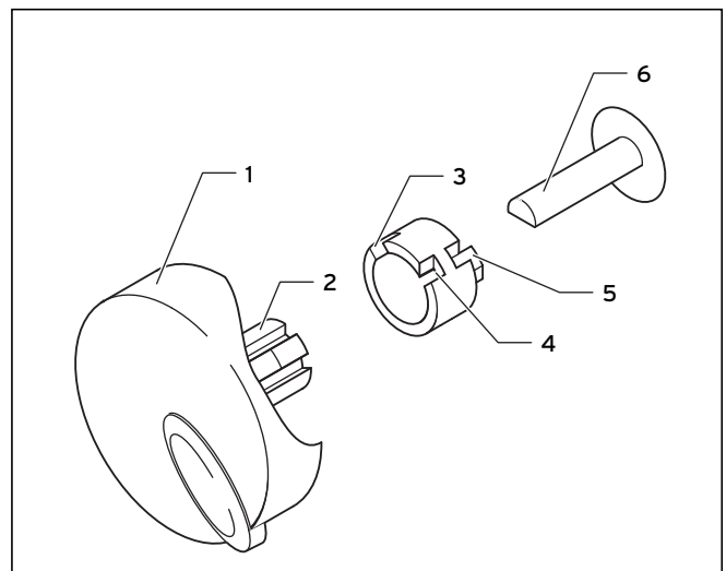
Fig. 9.1 Limitazione del campo di regolazione della temperatura
