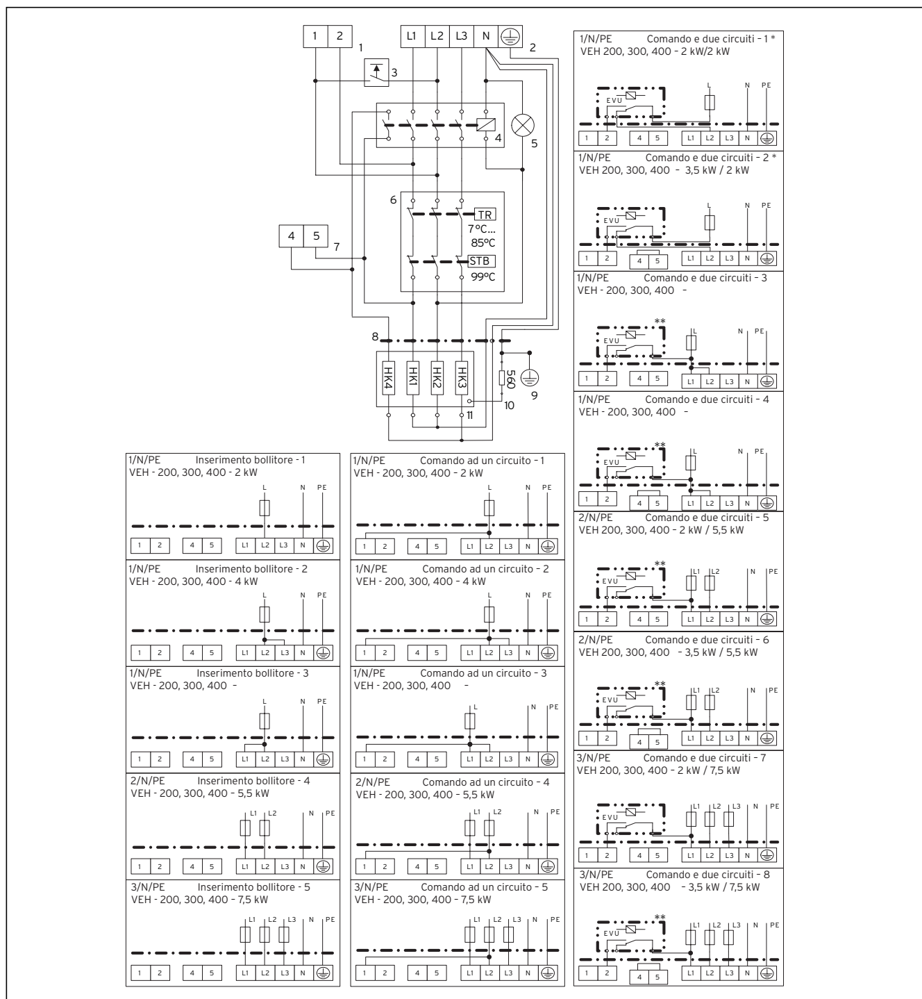
Fig. 8.1 Panoramica dei circuiti elettrici eloSTOR
