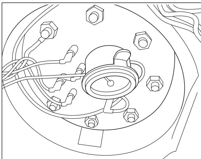
Abb. 7.14 Befestigen des Thermometers
