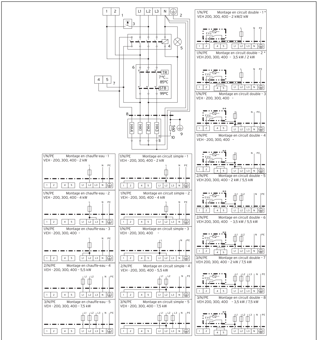
Fig. 8.1 Schéma de commutation Vue d'ensemble eloSTOR
