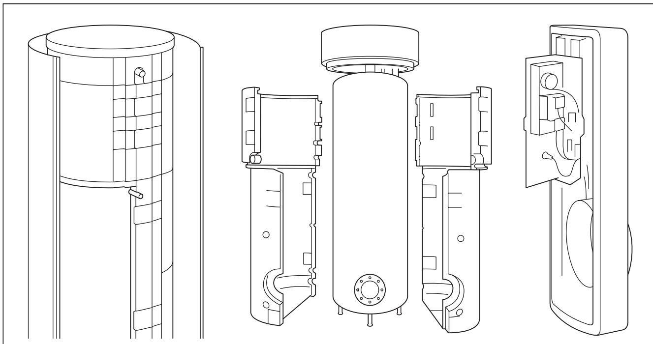
Abb. 2.1 Aufbau des Gerätes - Ummantelung (links), Isolierungskonzept (Mitte) und E-Box (rechts)
