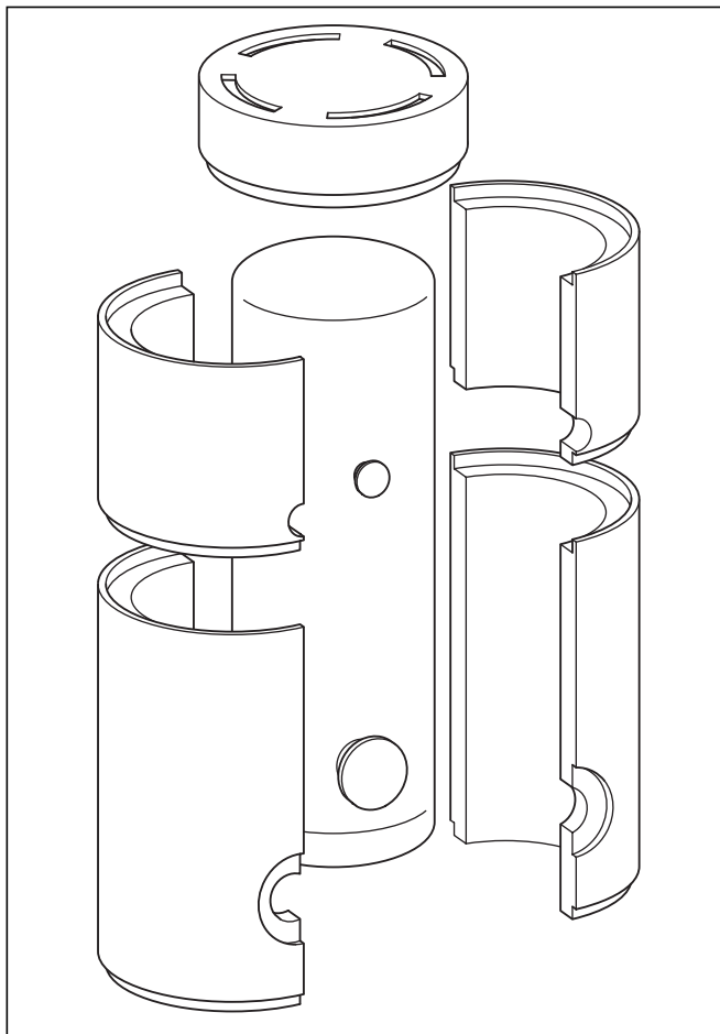
Fig. 7.18 Retrait de l'isolation
