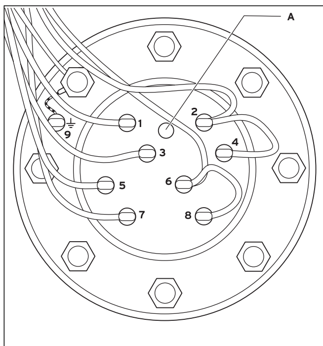
Fig. 8.13 Zone de commutation du collet de chauffage
