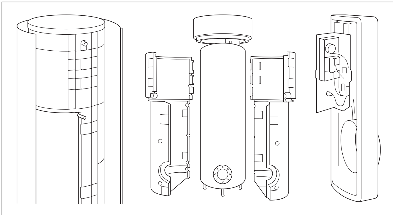
Fig. 2.1 Struttura dell'apparecchio - rivestimento (sinistra), tipo di isolamento (centro) e scatola elettrica (destra)
