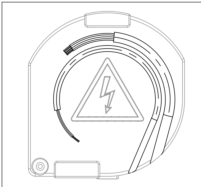
Fig. 8.12 Isolamento flangia con sagoma per accorciare il cavo
