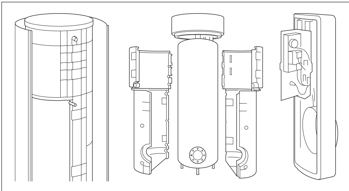
Fig. 2.1 Structure de l'appareil - Housse (gauche), concept d'isolation (milieu) et E-Box (droite)
