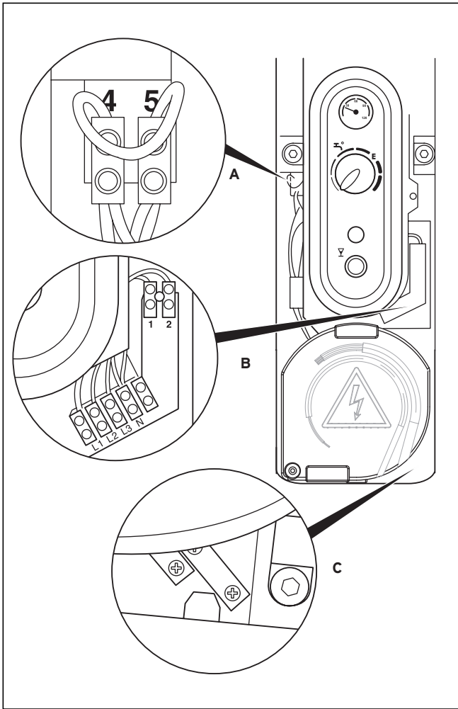
Abb. 8.5 Anschlusskasten
