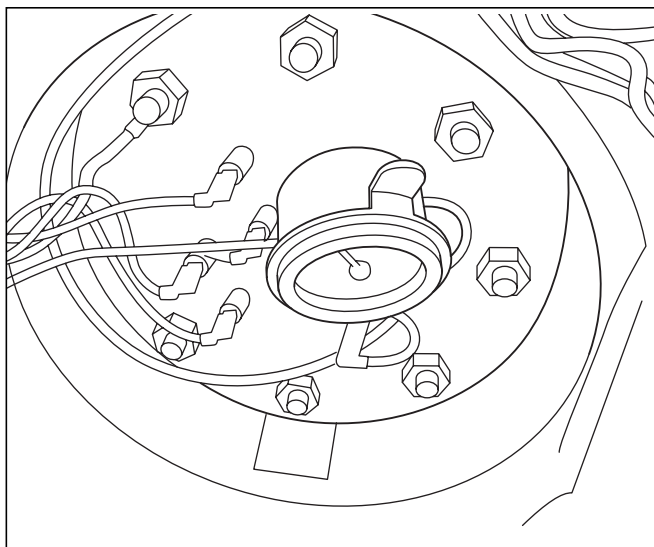
Fig. 7.14 Fixation du thermomètre
