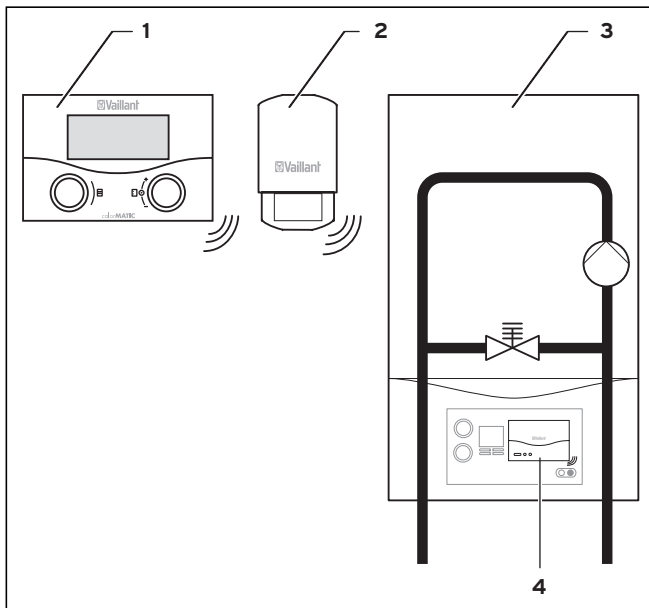
Abb. 2.1 Systemschema
