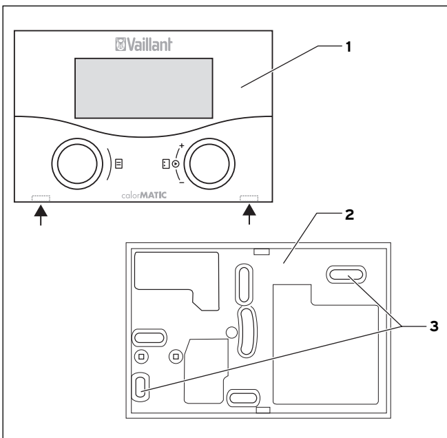
Abb. 4.6 Montage des colorMATIC 430f
