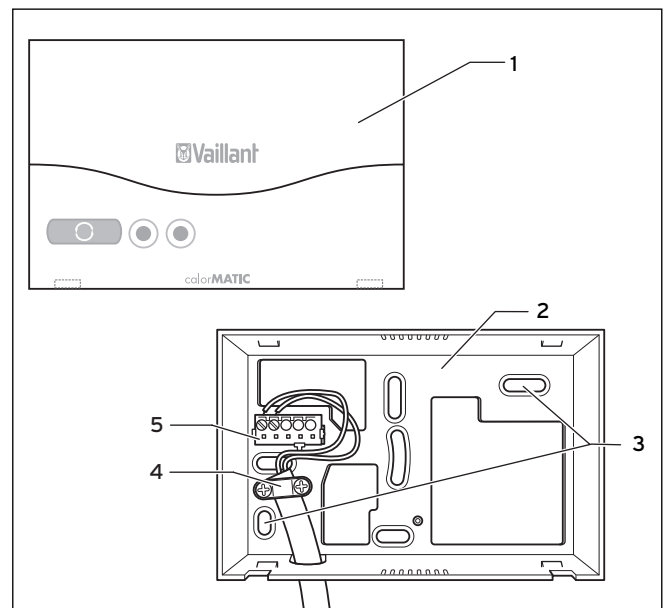
Abb. 4.1 Montage der Funkempfängereinheit
