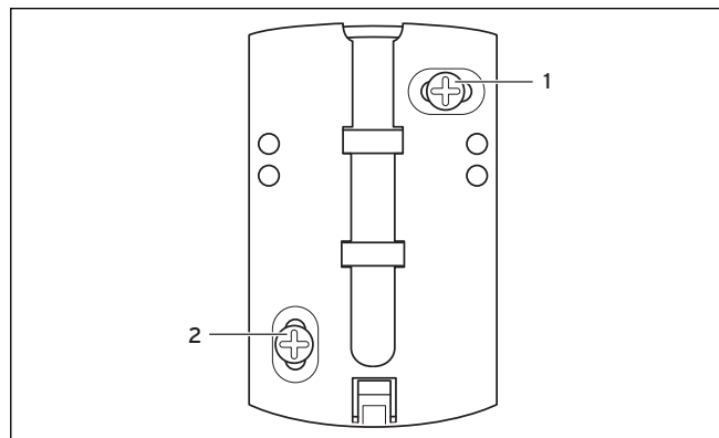
Abb. 4.3 Wandhalter montieren
