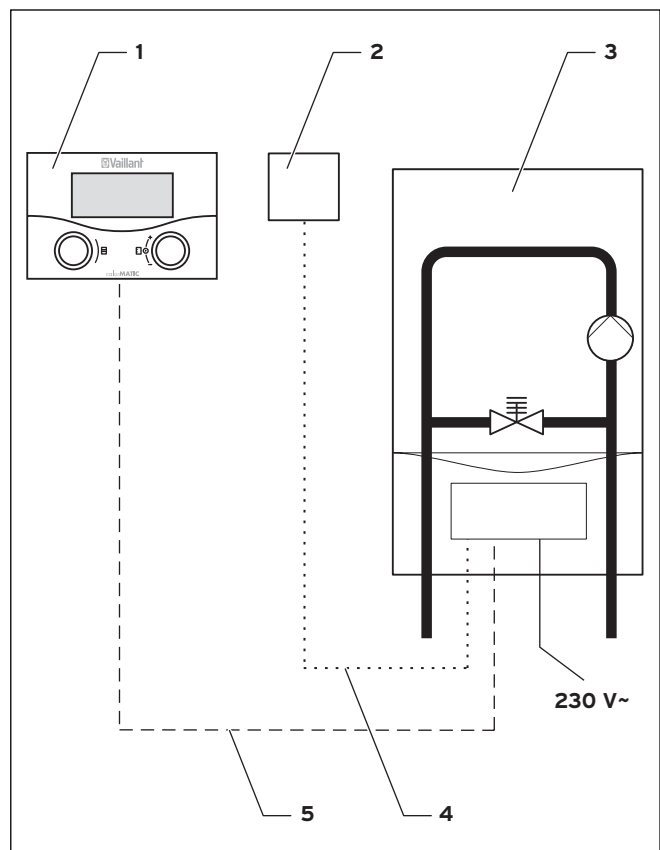
Abb. 2.1 Systemschema
