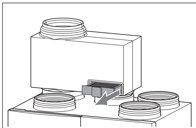
Abb. 6.2 Bypass-Filter entnehmen
