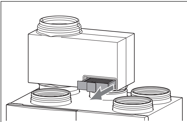
Abb. 6.2 Bypass-Filter entnehmen
