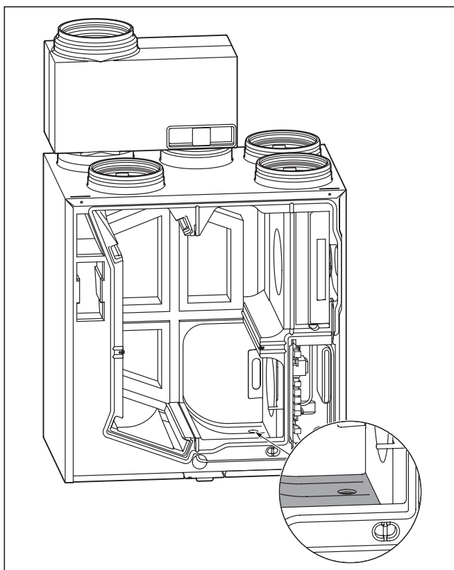
Abb. 6.2 Kondenswasserabfluss
