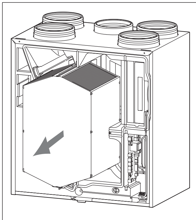
Abb. 6.1 Wärmetauscher ausbauen
