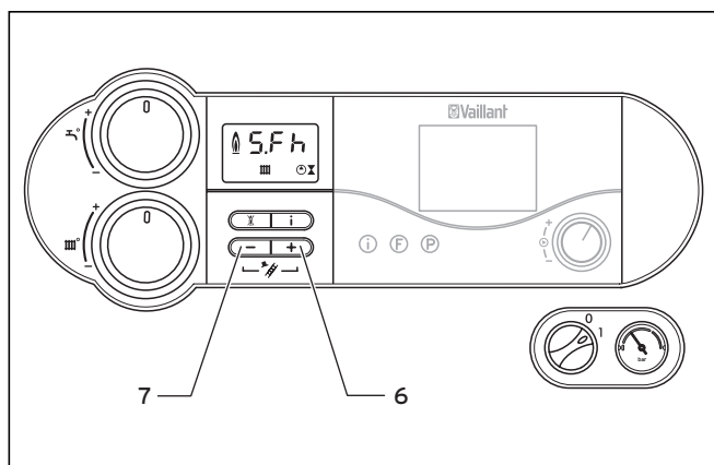
Abb. 4.16 Schornsteinfeger-Betrieb einschalten
