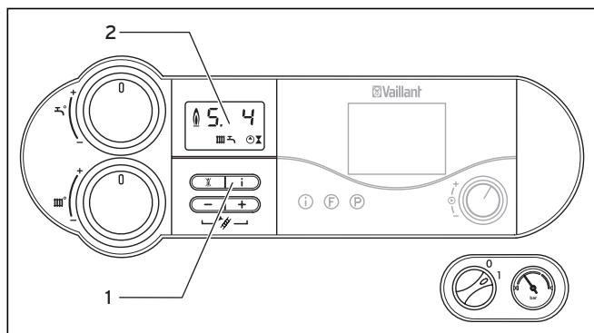
Abb. 4.11 Statusanzeigen
