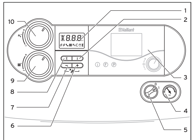
Abb. 4.2 Bedienelemente
