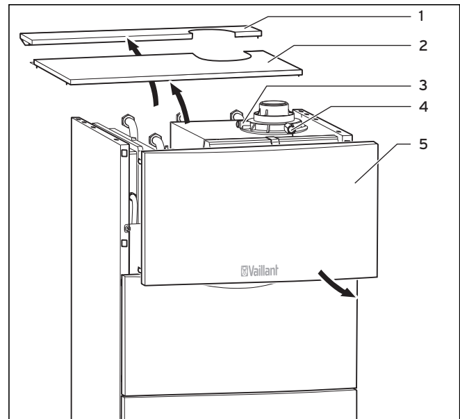
Abb. 4.15 Schornsteinfeger-Messung
