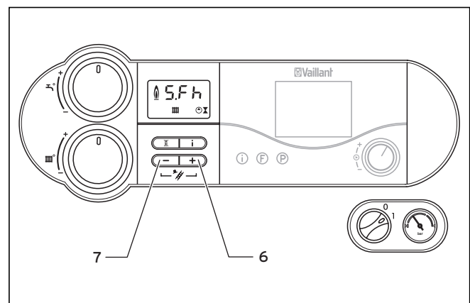
Abb. 4.16 Schornsteinfeger-Betrieb einschalten
