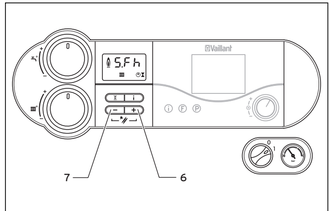
Abb. 4.16 Schornsteinfeger-Betrieb einschalten
