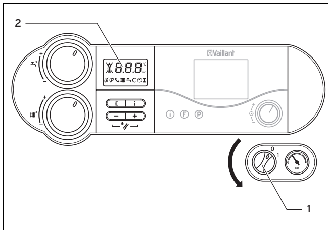
Abb. 4.14 Gerät ausschalten
