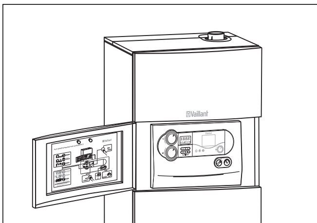
Abb. 4.1 Verkleidungstür öffnen
