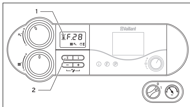
Abb. 4.12 Entstörung
