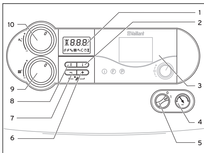
Abb. 4.2 Bedienelemente
