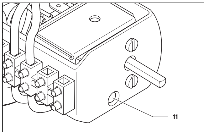
Slika 4 Pozicija bezbednosne temperaturne sklopke
