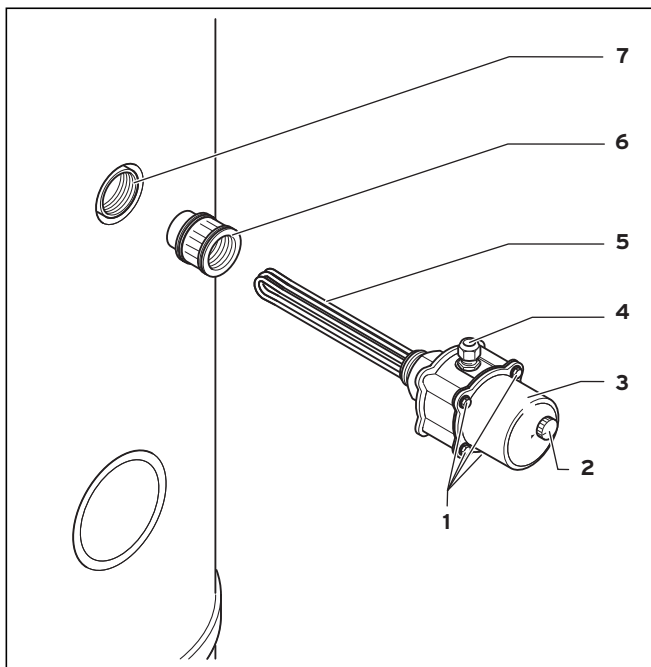
Abb. 1 Elektroheizstab installieren
