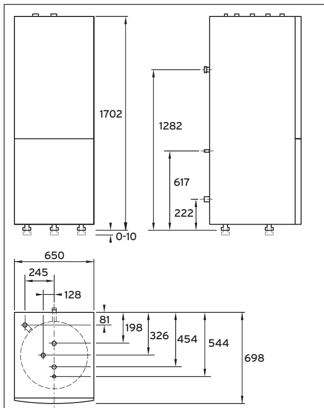
Abb. 4.2 Abmessungen
