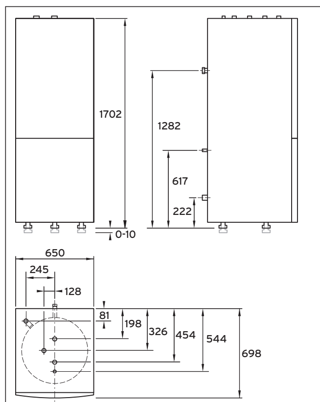
Fig. 4.2 Dimensions
