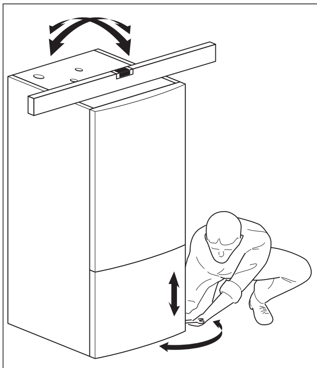
Bild 4.3 Rikta apparaten
