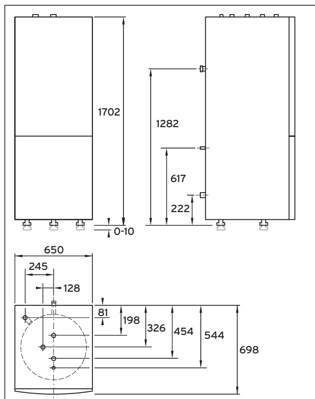
Afb. 4.2 Afmetingen
