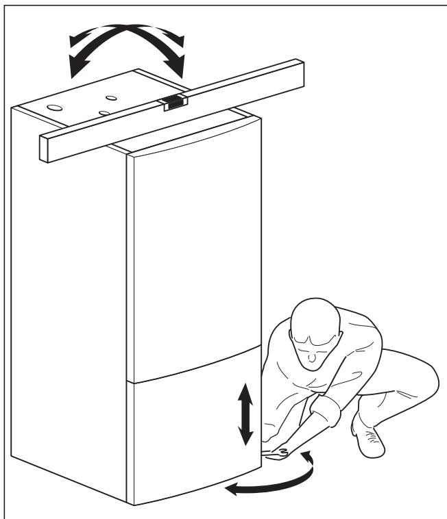
Abb. 4.3 Gerät ausrichten
