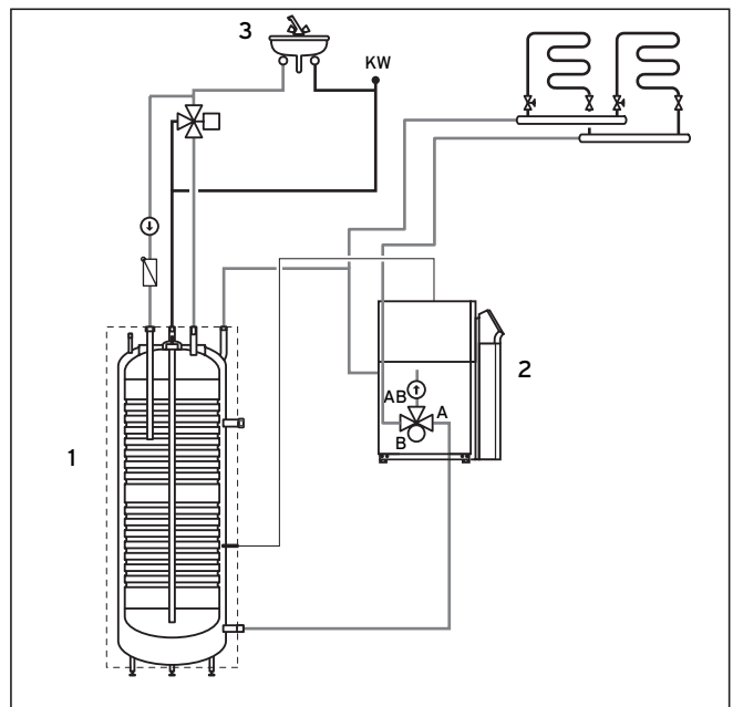
Kuva 4.4 Asennus lämminvesivaraajaksi ilman lämmityspattereita
