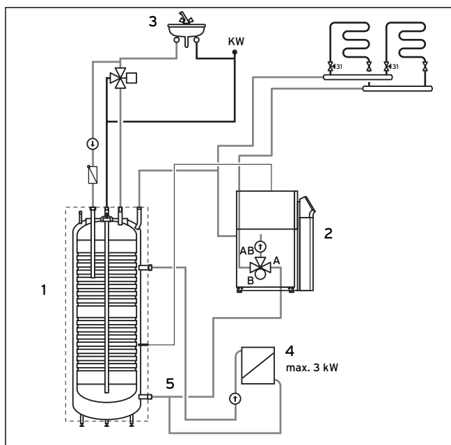
Afb. 4.5 Installatie als warmwaterboiler met extra radiator
