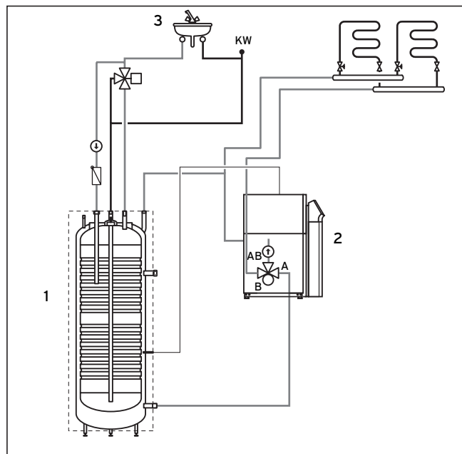
Abb. 4.4 Installation als Warmwasserspeicher ohne Radiatorheizkörper
