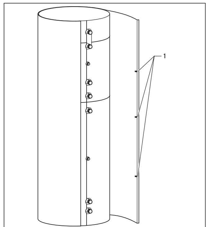
Abb. 5.9 Verkleidungsmantel lösen
