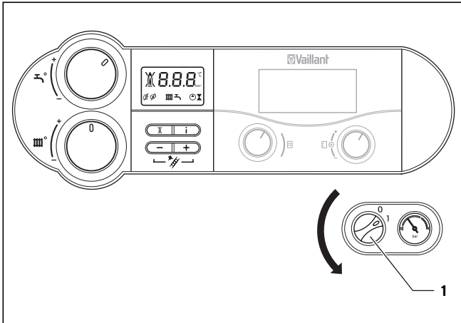
Abb. 5.18 Gerät ausschalten
