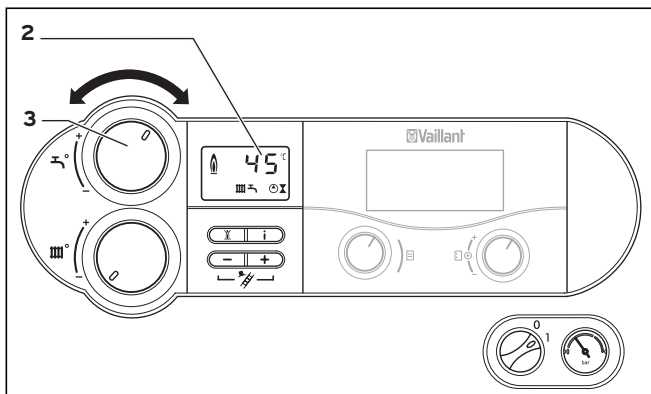
Abb. 5.11 Warmwassertemperatur einstellen
