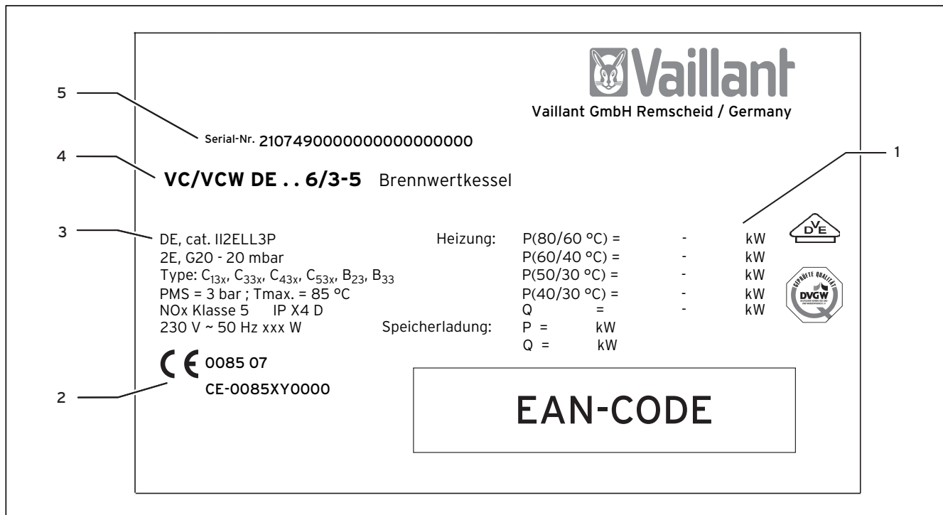
Abb. 1.1 Typenschild
