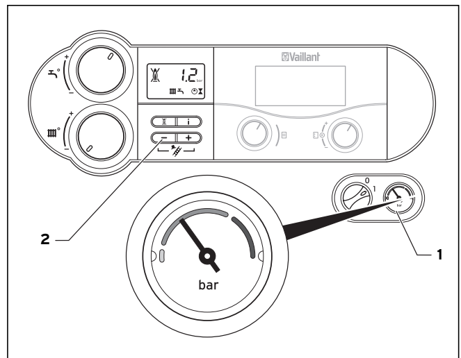
Abb. 5.17 Heizungsanlage füllen
