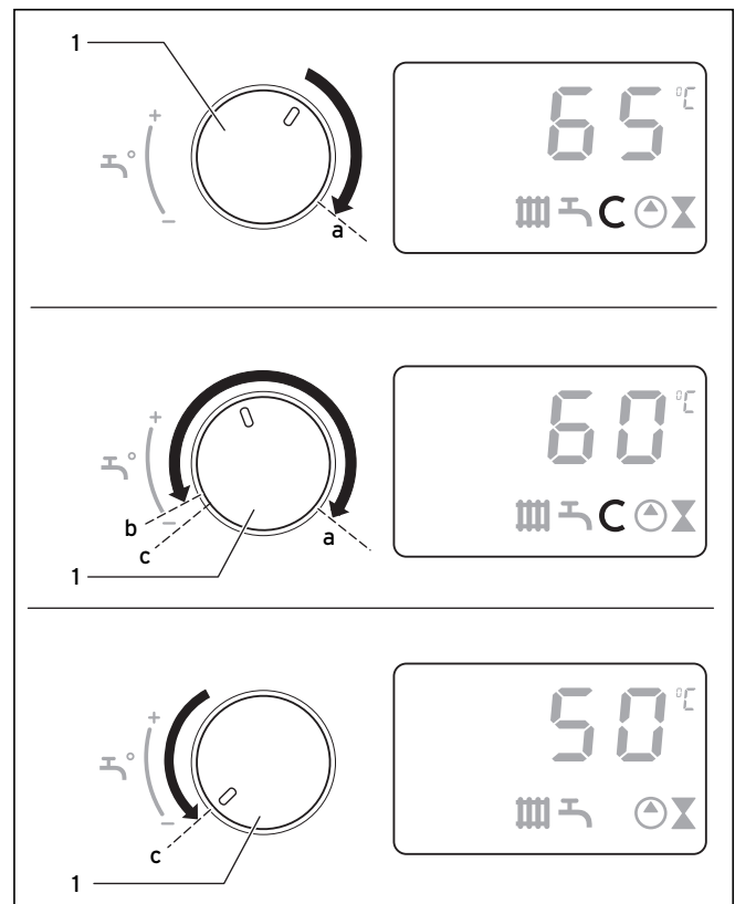
Abb. 5.8 Einstellbereich für die Speichertemperatur
