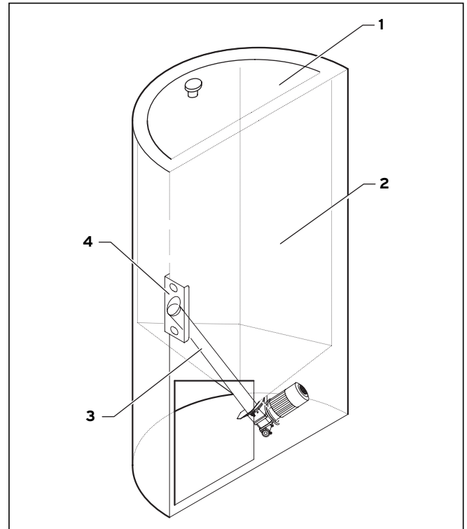
Abb. 5.7 Funktionselemente des Vorratsbehälters für Handbeschickung
