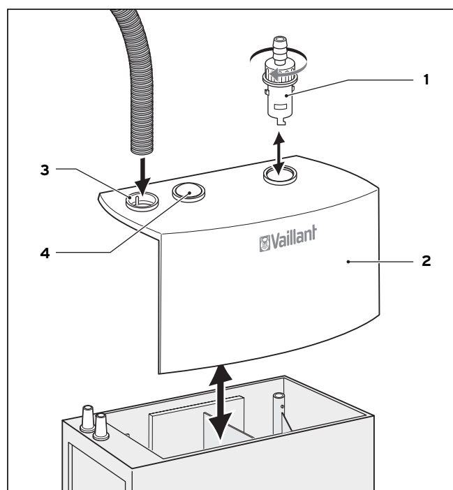
Fig. 5.1 Démontage du clapet anti-retour et du couvercle
