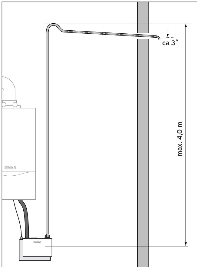
Abb. 5.2 Verlegung des Auslaufschlauchs
