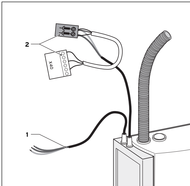
Rys. 6.1 Przegląd przyłączy elektrycznych
