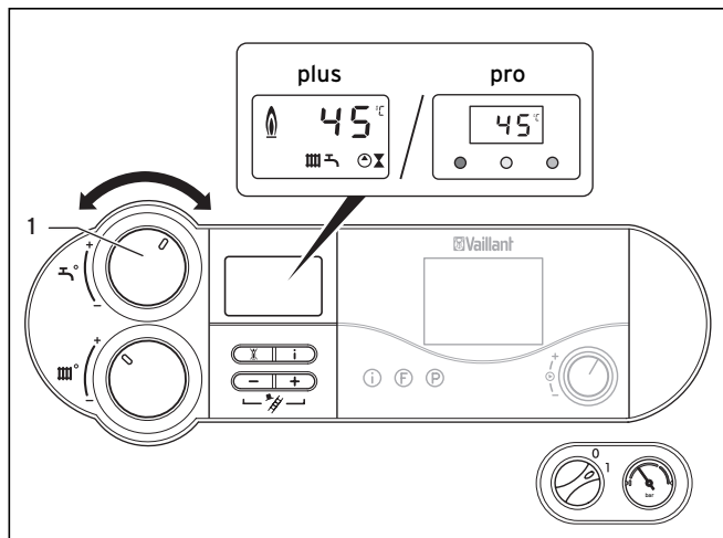
Afb. 4.1 Watertemperatuur instellen (voorbeeld: ecoTEC pro)
