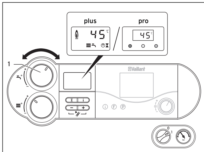
Abb. 4.1 Wassertemperatur einstellen (Beispiel: ecoTEC pro)
