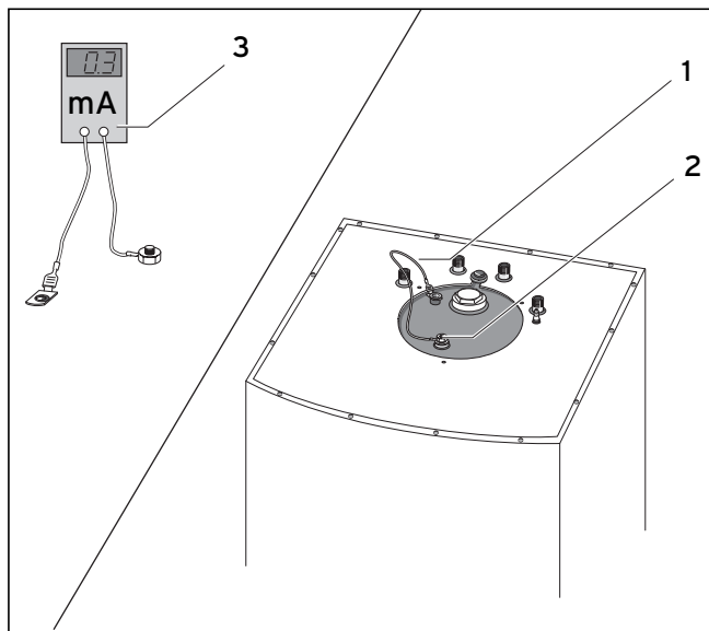
Abb. 7.1 Wartung der Schutzanode
