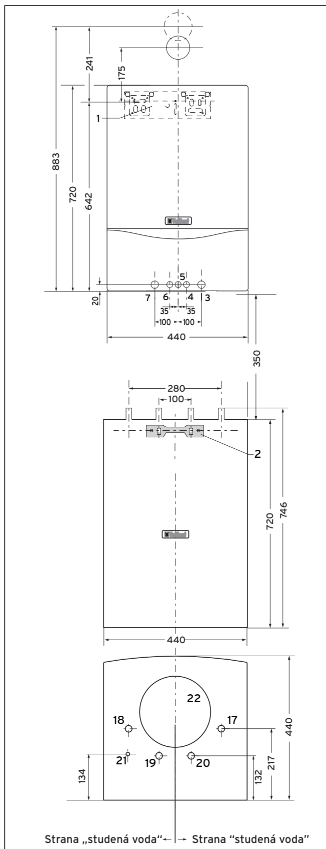
Obr. 4.3 Rozměry při montáži pod topným zařízením
