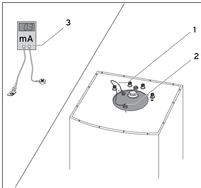
Abb. 7.1 Wartung der Schutzanode
