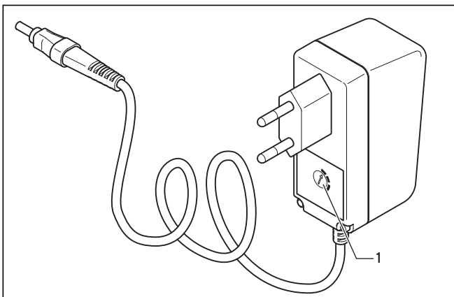
Abb. 4.2 Steckernetzteil des VPI-Displays/2
