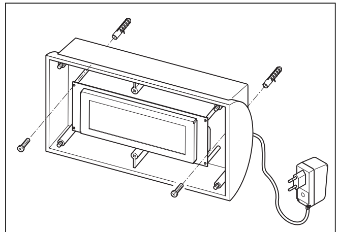
Abb. 6.2 VPI-Display/2 montieren
