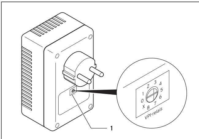
Abb. 6.4 Funkrelais für VPI-Display (Bsp.: Einstellung auf Kanal 0)
