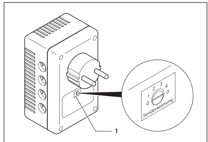
Abb. 6.5 Senderkennung am VPI-Adapter einstellen (Bsp.: Einstellung auf Kanal 0)
